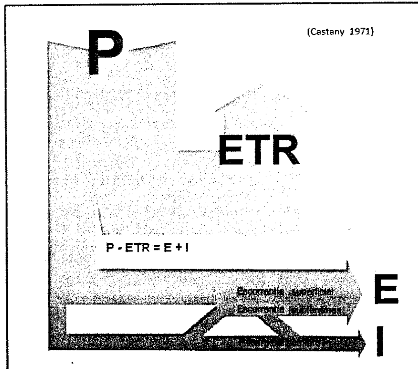
Figura 3. Esquema tomado del Libro Blanco del Agua ( Ministerio de Medio Ambiente, 2001 ) y del Plan Hidrológico del Júcar 2009-2015 con las componentes del ciclo hídrico ( Castany, 1971 )
