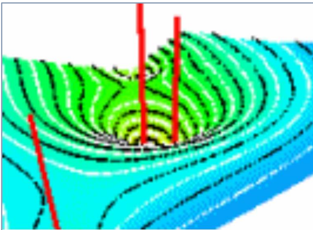
Figura 46 Instantánea de la modelización de la interacción de varios conos de bombeo originados por varios pozos en explotación (líneas rojas). Fuente: Instituto Federal de Geociencias y Recursos Naturales de Alemania en www.bgr.bund.de
