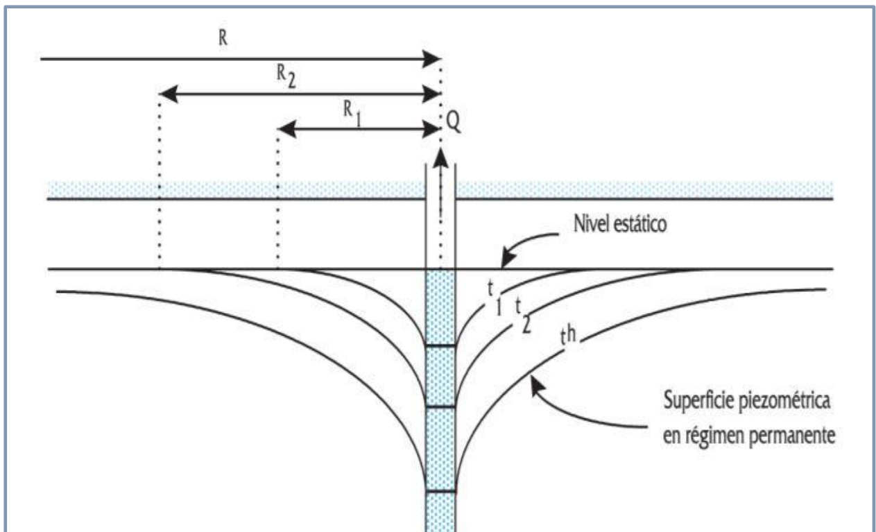
Figura 44 Evolución del cono de descensos en un pozo de bombeo y de su radio de influencia a lo largo del tiempo. Fuente: Universidad Politécnica de Cataluña. https://www.upc.edu/ca
