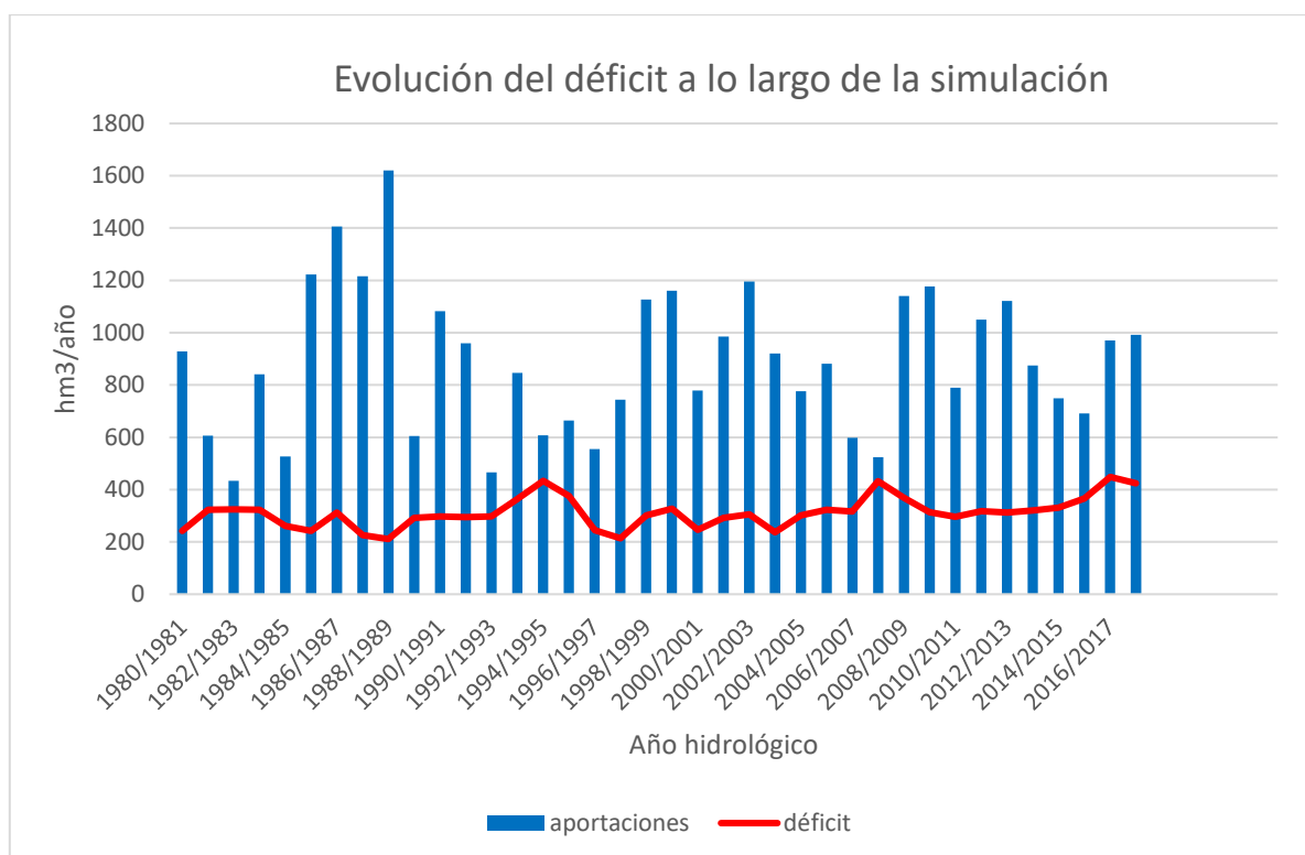
Figura 3. Evolución del déficit a lo largo de la simulación. Horizonte 2021. Periodo 1980/81-2017/18. ATS aplicando las vigentes reglas de explotación 1980/81-2017/18, 295 hm³/año
