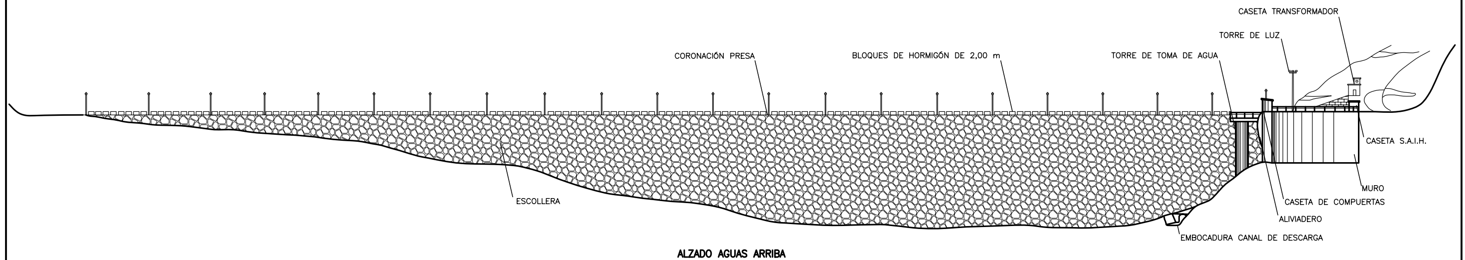
ALZADO AGUAS ARRIBA
