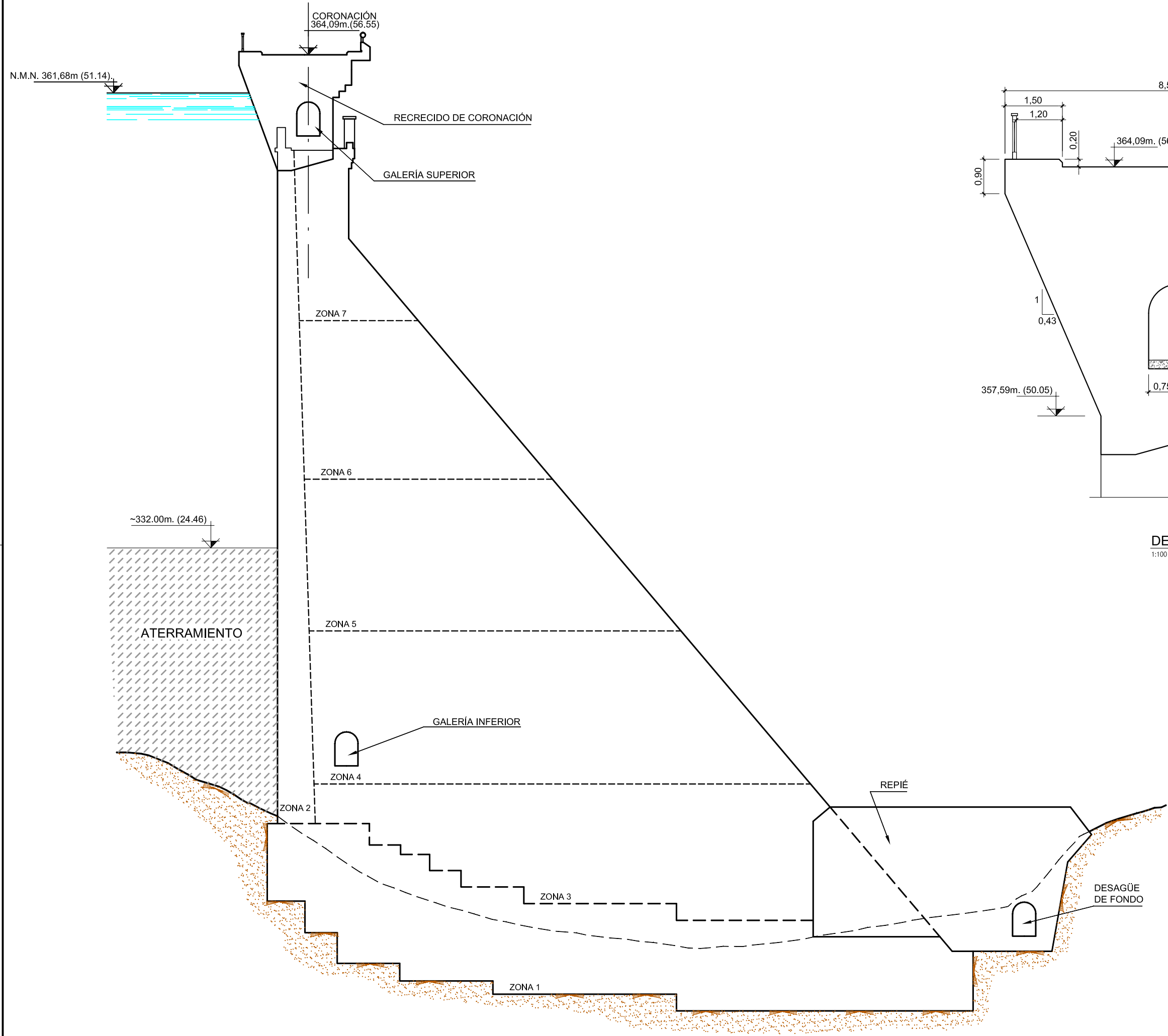
SECCIÓN TIPO 1:250
