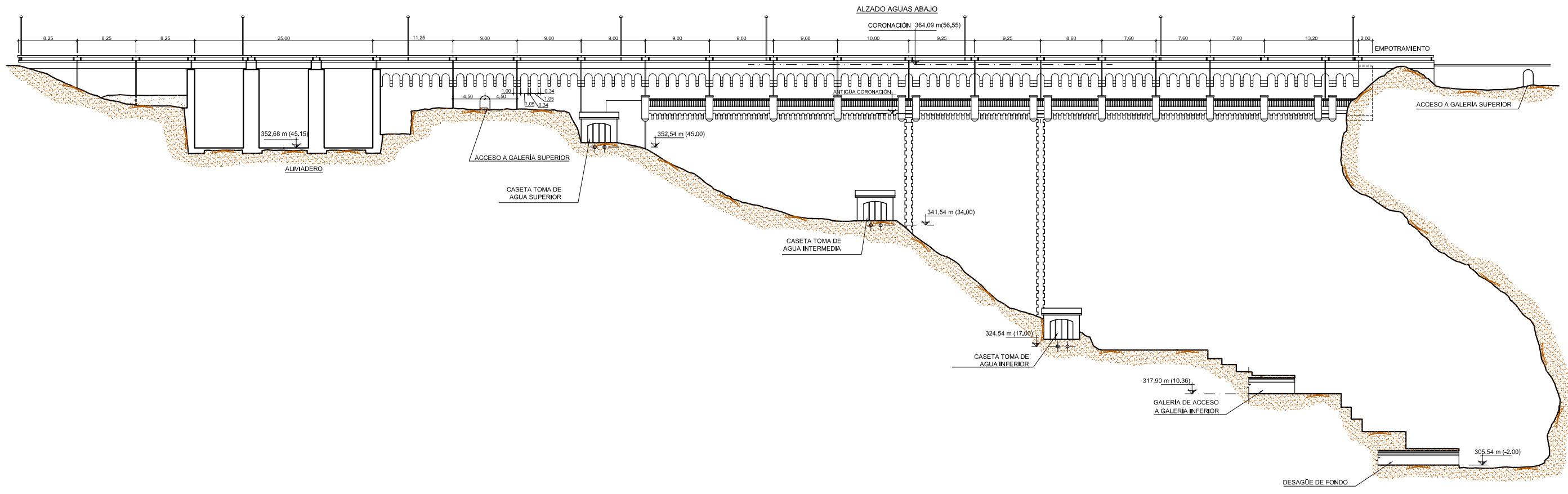
ALZADO AGUAS ABAJO 1:500
