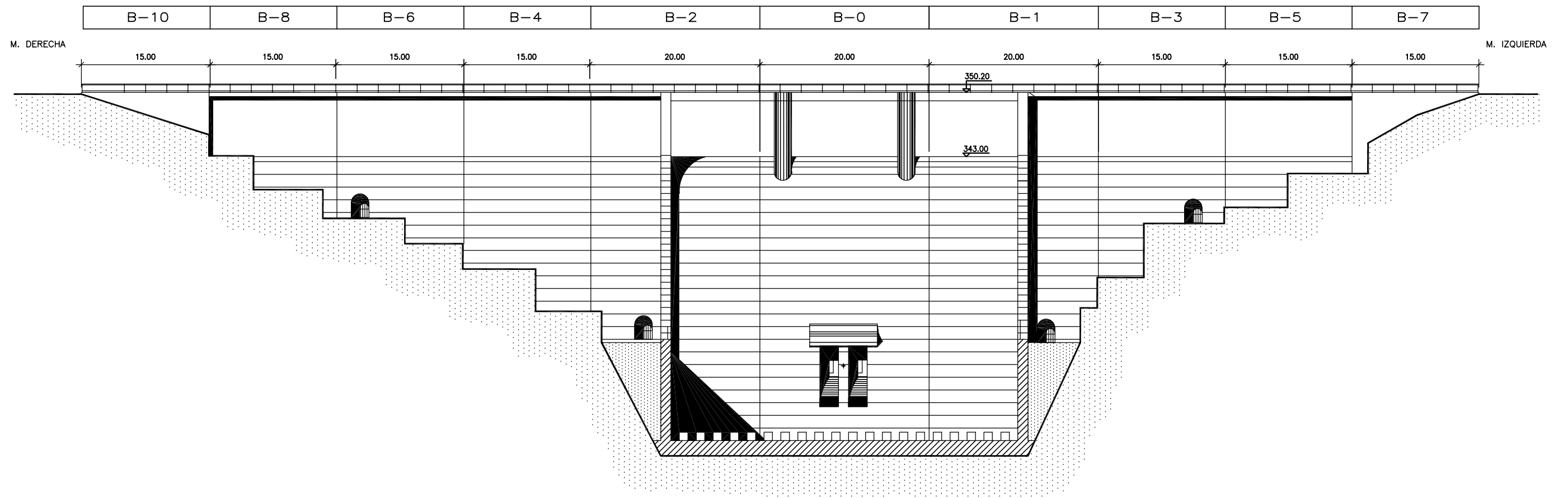
ALZADO AGUAS ABAJO
