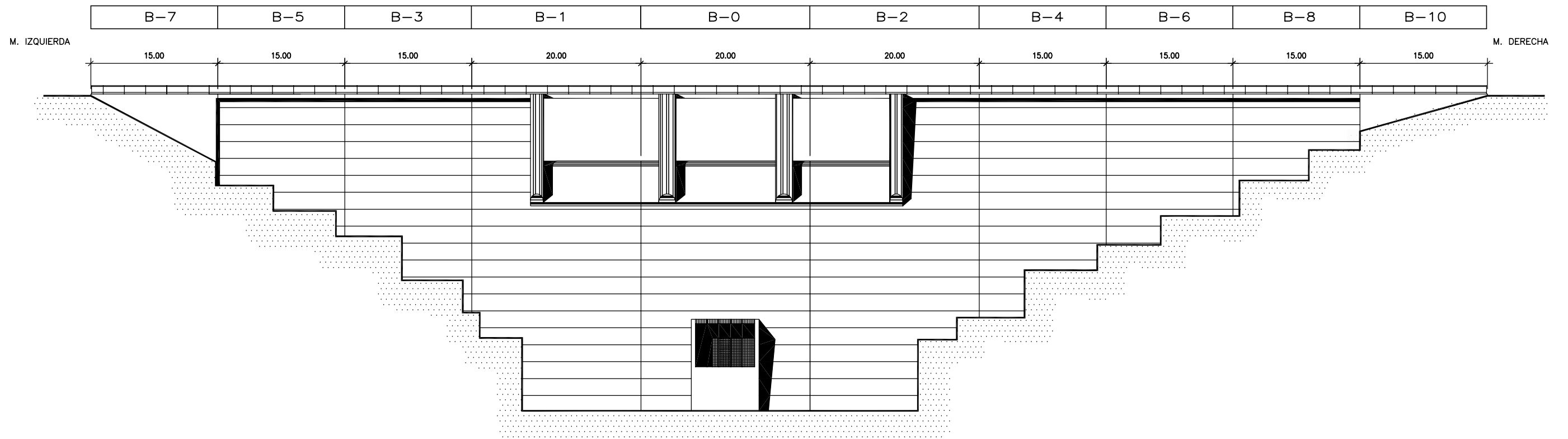
ALZADO AGUAS ARRIBA
