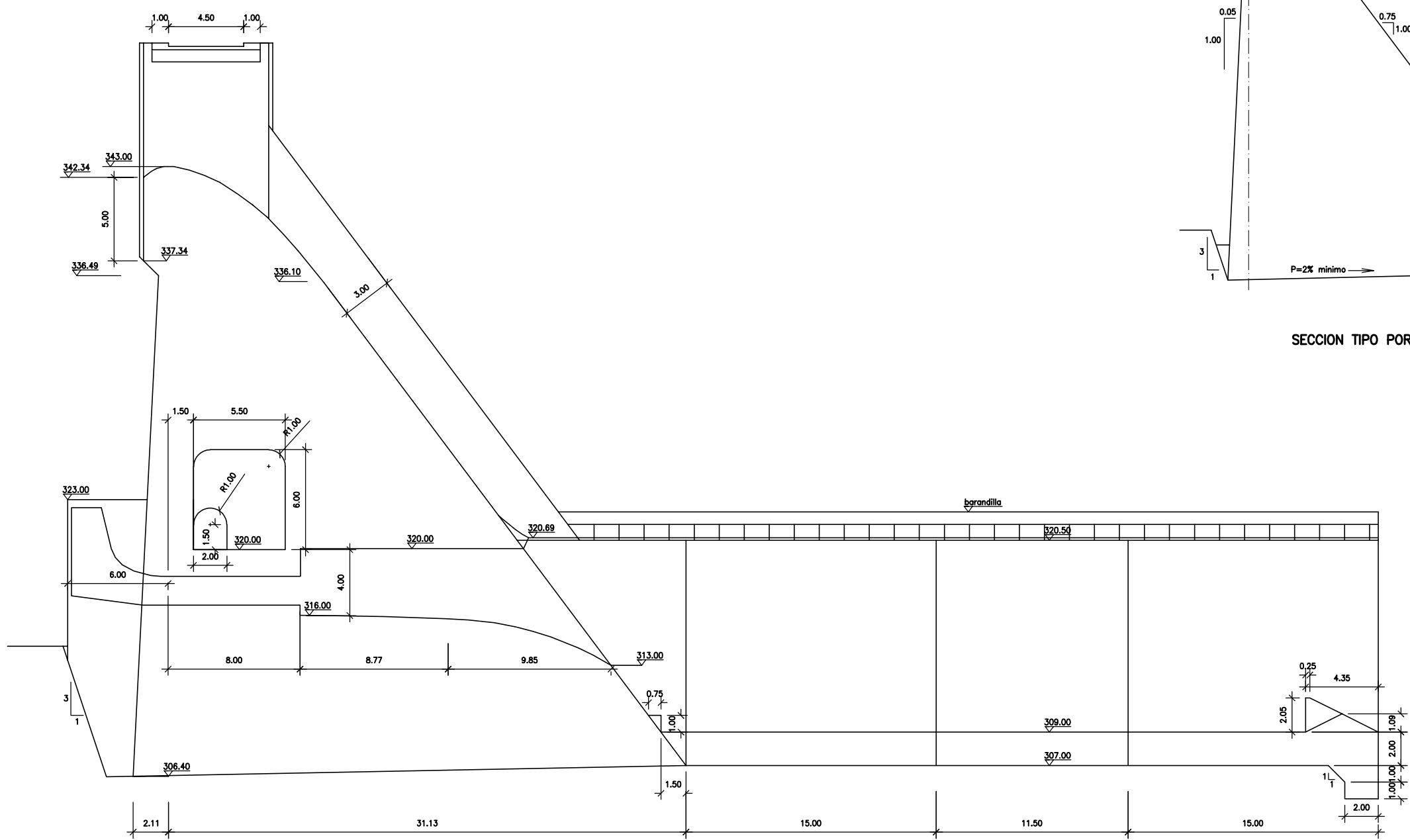
SECCION TIPO POR ALMADERO
