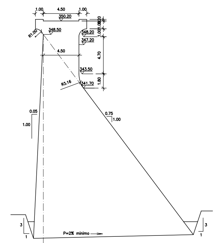
SECCION TIPO POR ESTRIBOS
