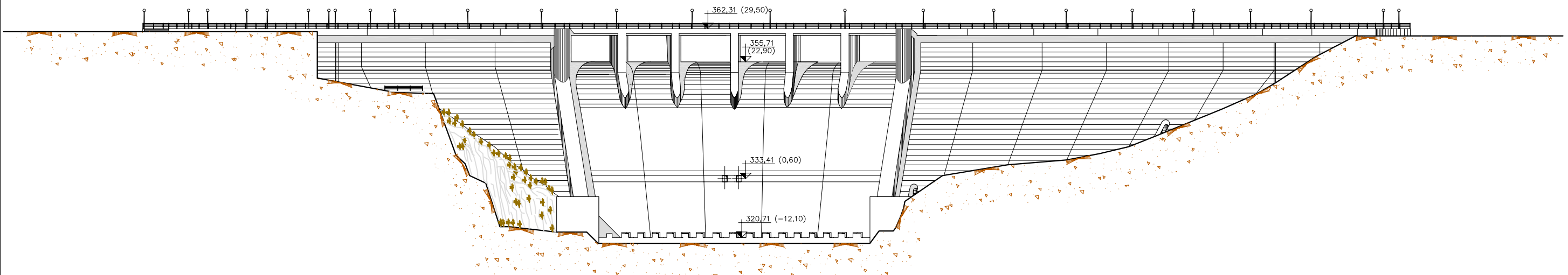
ALZADO AGUAS ABAJO ESCALA 1:1000
