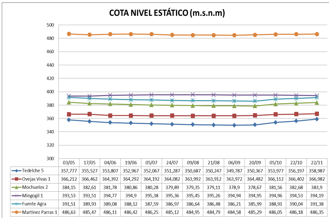
Figura 2. Evolución cota nivel estático en los sondeos en explotación BES Hellín.
