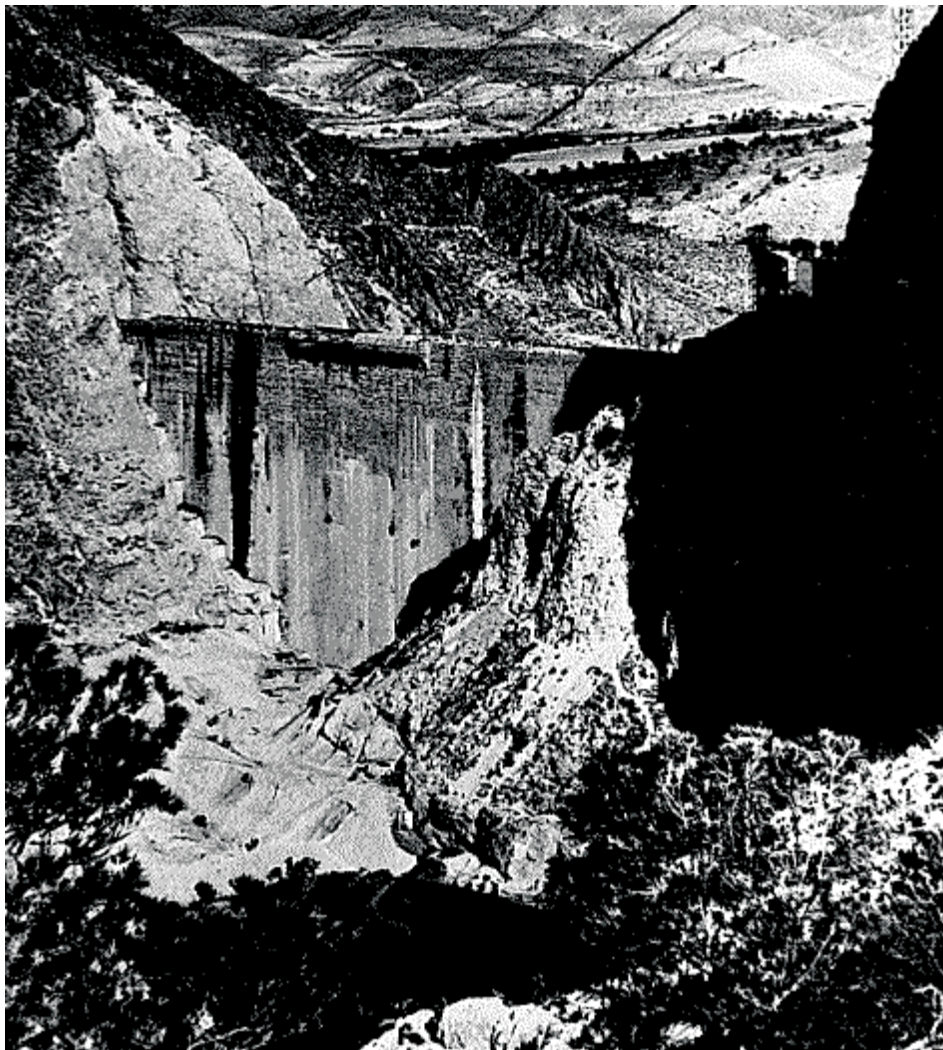
Paramento de la presa aguas arriba (1959).
