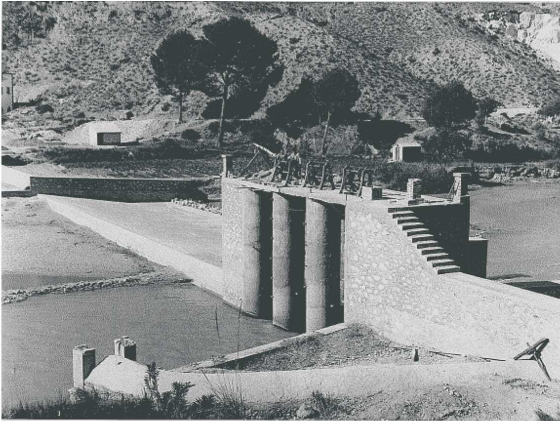
Presa de derivación para reposición de los riesgos tradicionales.
