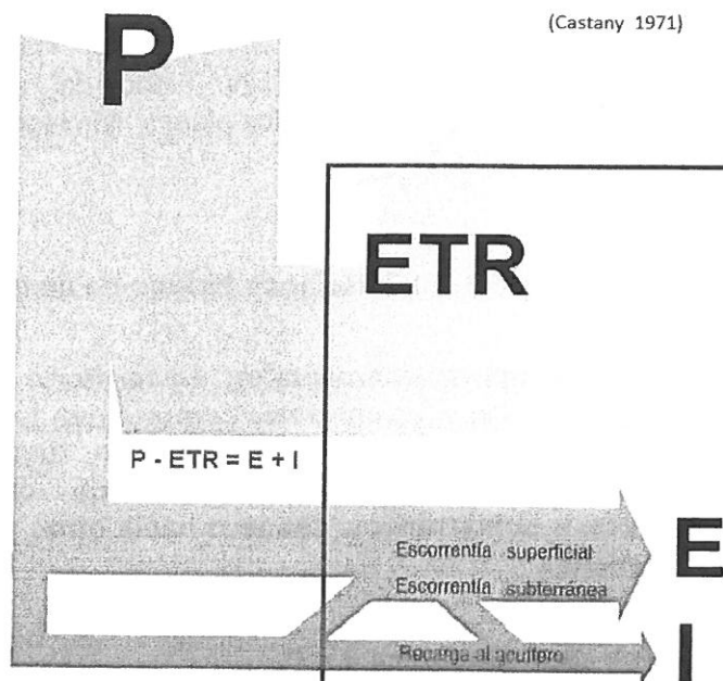
Figura 3. Esquema tomado del Libro Blanco del Agua (Ministerio de Medio Ambiente, 2001) y del Plan Hidrológico del Júcar 2009-2015 con las componentes del ciclo hídrico (Castany, 1971)
