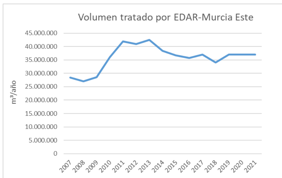
Figura 6 Volumen tratado por la EDAR Murcia Este entre los años 2007-2021.
