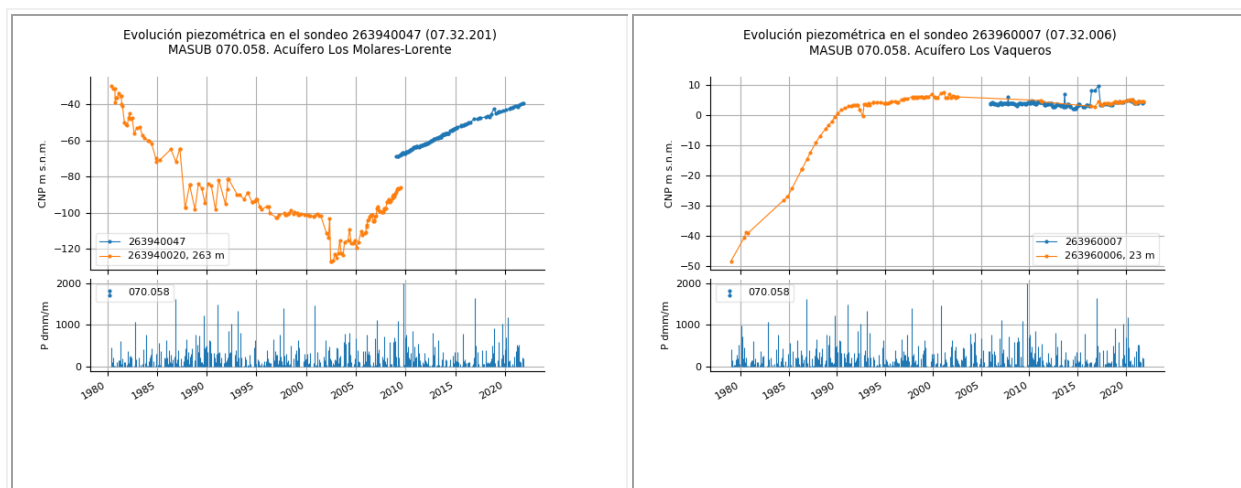
Figura 32 Evolución piezométrica en el acuífero Los Vaqueros y acuífero Los Morales-Lorente. MASub 070.058
