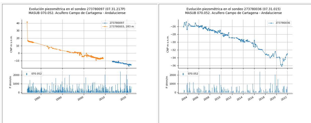
Figura 27 Evolución piezométrica del acuífero Andaluciense de la MASub 070.052 Campo de Cartagena
