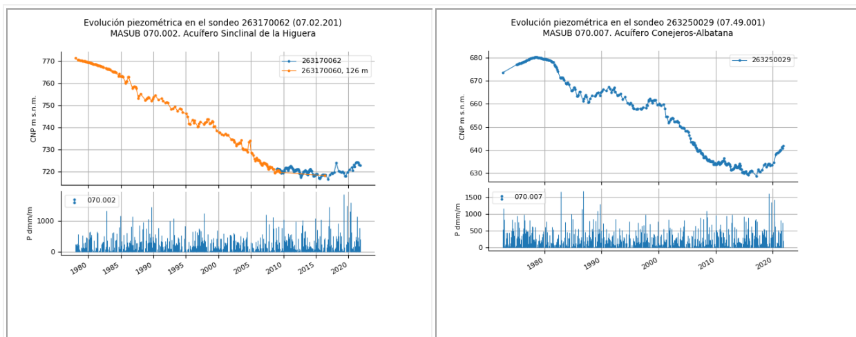
Figura 19 Evolución piezométrica en el acuífero Sinclinal de la Higuera-MASub 070.002-
