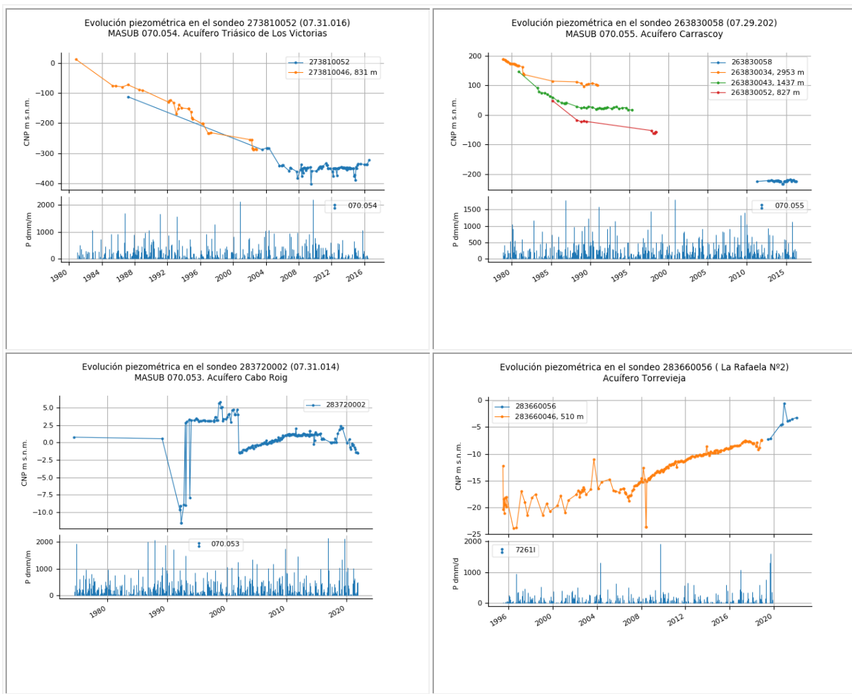
Figura 29 Evolución piezométrica en las MASUB 070.054 Triásico de Los Victorias y 070.055 Triásico de Carrascoy, 070.053 Cabo Roig y 070.042 Terciario de Torreveja (Gráfica del punto de control de la DPA)
