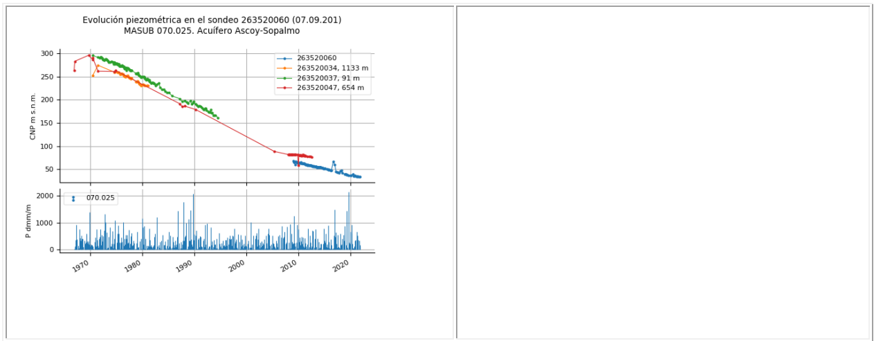
Figura 20 Evolución piezométrica en MASub del Altiplano (Gráfica MASub 070.027 Serral Salinas. Fuente: DPA).
