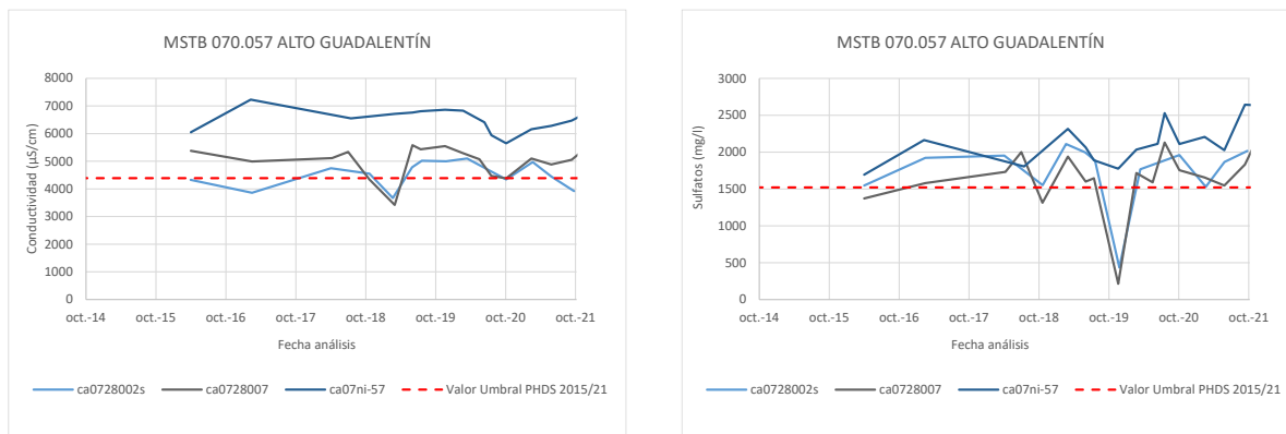
Figura 41 Evolución de la concentración media de cloruros, conductividad y sulfatos y evolución de los incumplimientos de cloruros, conductividad y sulfatos en la MASUB 070.057 Alto Guadalentín.
