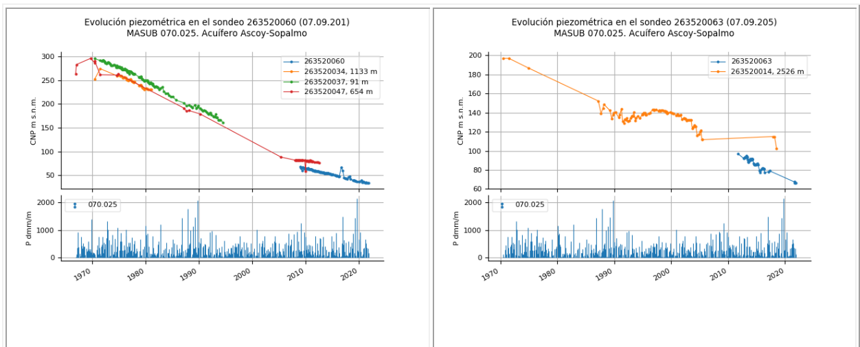
Figura 21 Evolución piezométrica en acuíferos de las MASub 070.025 Ascoy-Sopalmo
