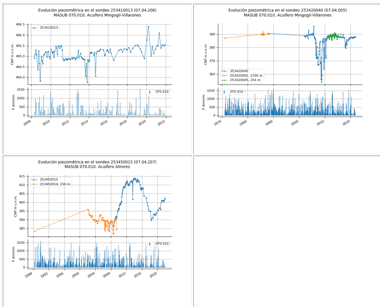
Figura 13 Evolución piezométrica en el acuífero Mingogil-Villarones y Almirez de la MASub 070.010.
