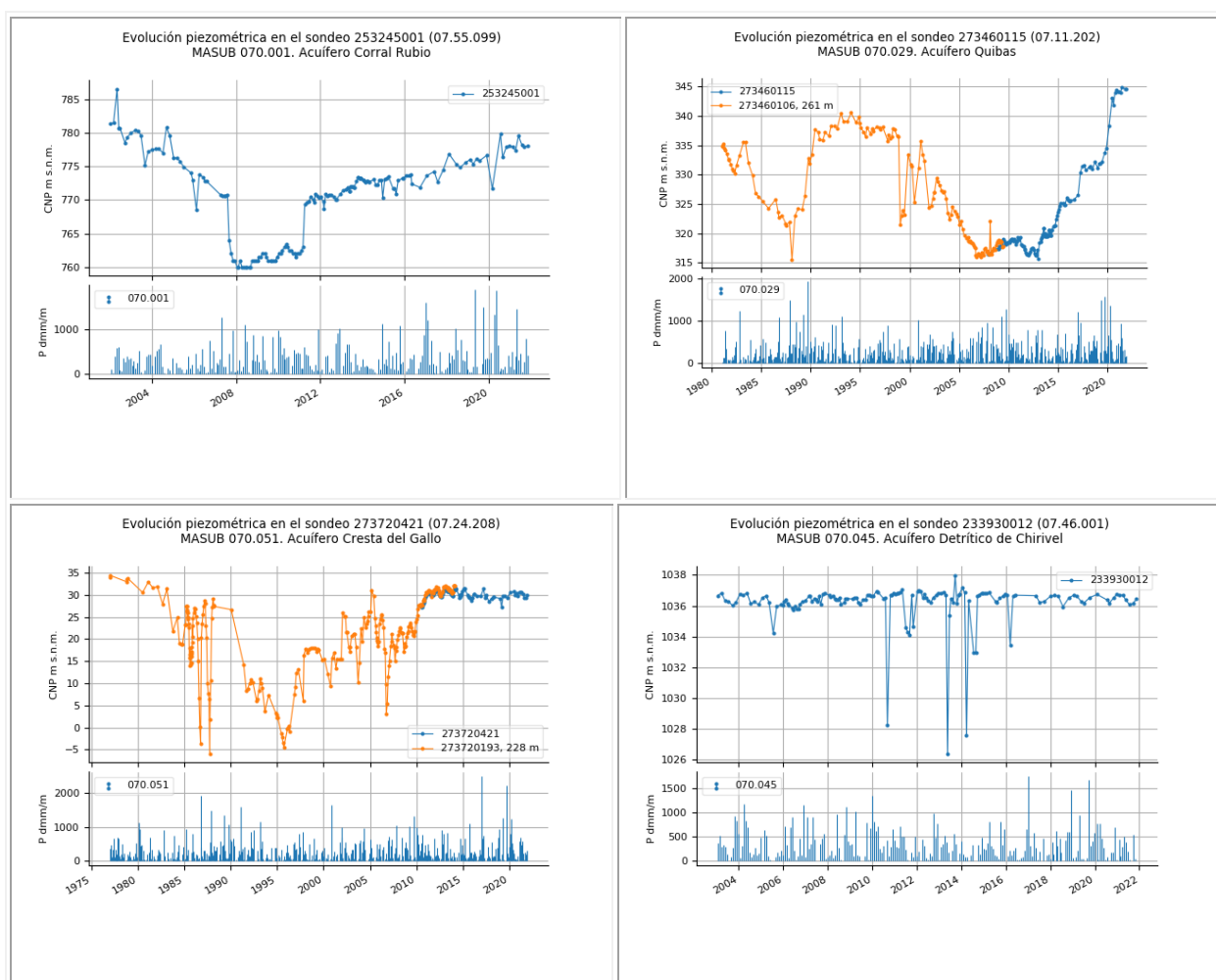
Figura 31 Evolución piezométrica en MASub que han mejorado su estado cuantitativo
