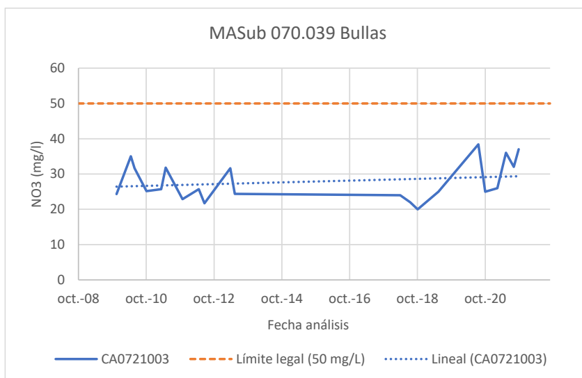
Figura 38 Evolución de puntos de control que presentan incumplimiento por concentraciones de nitratos en el año 2021 en la masa de agua subterránea 070.039 Bullas (acuífero Bullas).
