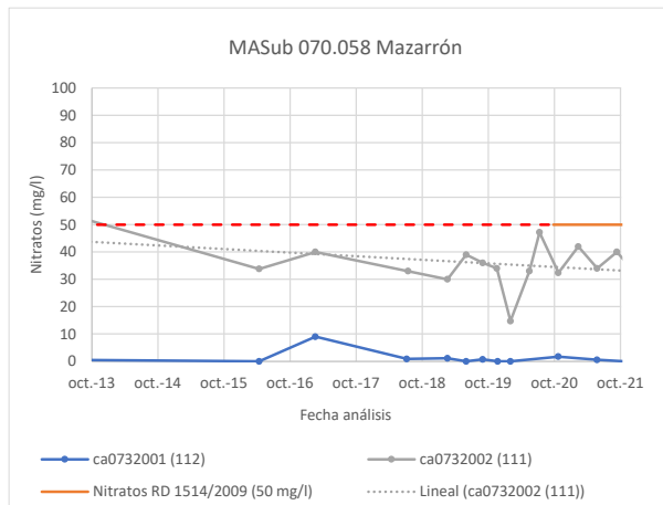
Figura 46 Evolución de la concentración de nitratos en las masas de agua subterránea que mejora su estado químico en el año 2021.
