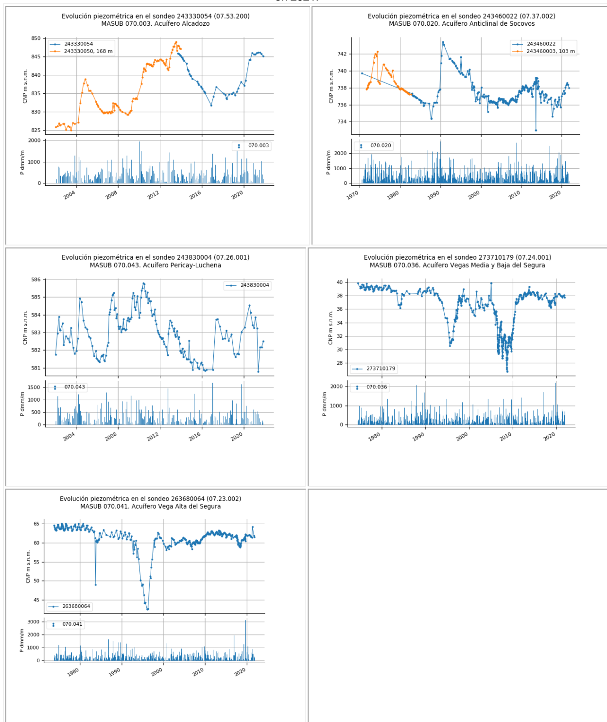
Figura 30 Evolución piezométrica en acuíferos de MASub en Buen Estado cuantitativo en el año 2021.
