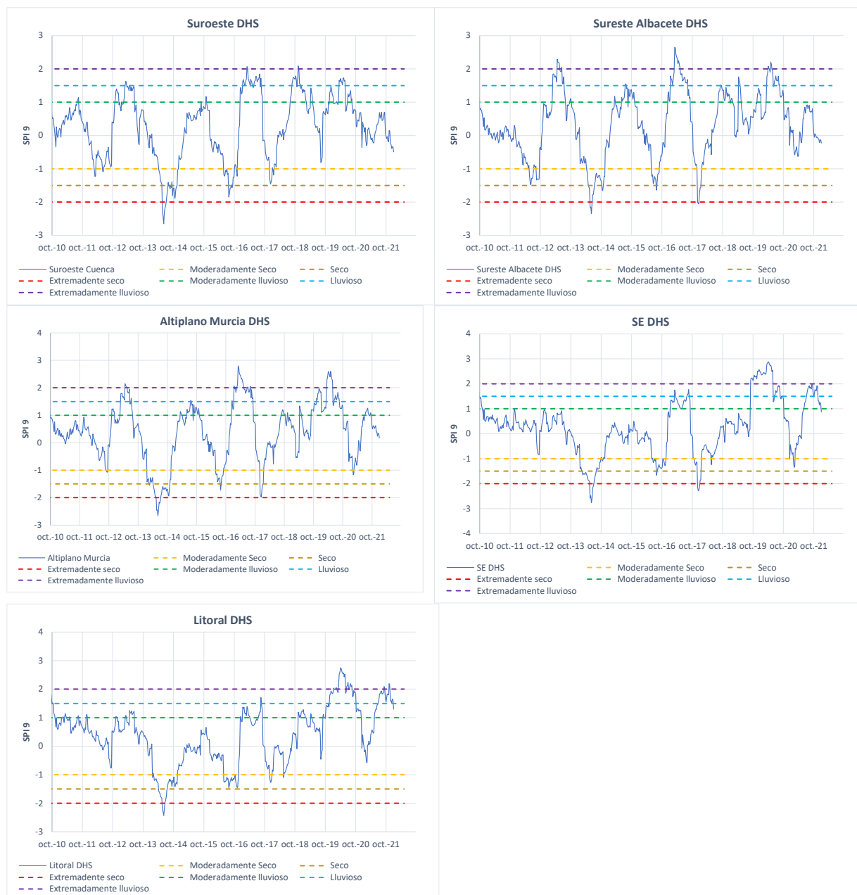
Figura 12 Evolución del índice SPI en puntos seleccionados de la demarcación
