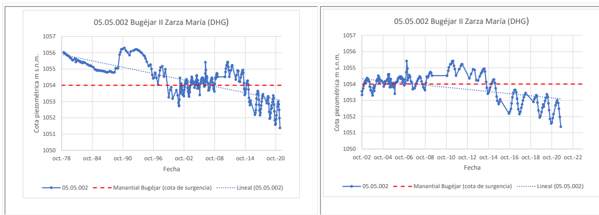
Figura 17 Evolución piezométrica en el acuífero compartido La Zarza-Bujéjar. MASub 05.05 La Zarza (DHG).
