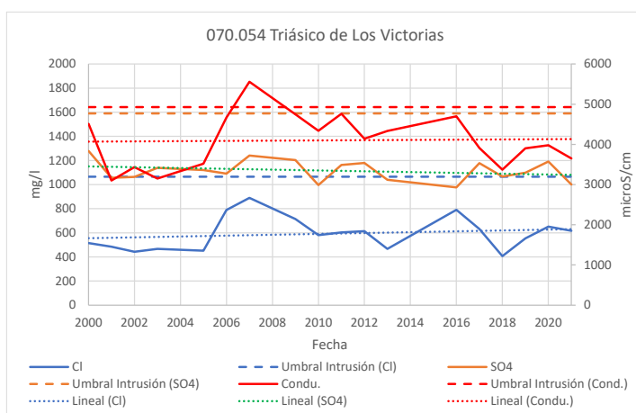
Figura 44 Evolución de punto de control que presenta incumplimiento por conductividad en el año 2020 en la masa de agua subterránea 070.054 Triásico de Los Victorias.
