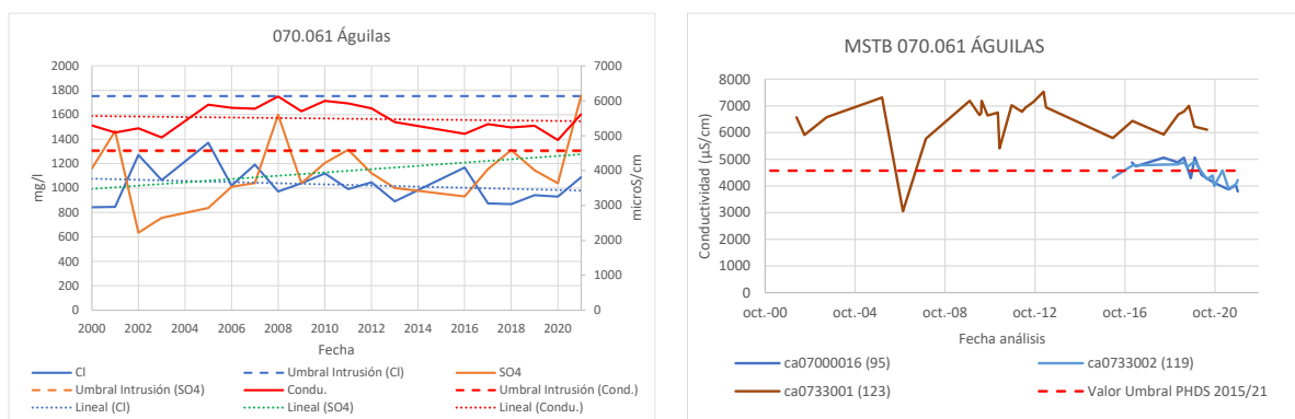
Figura 43 Evolución de la concentración media de cloruros, conductividad y sulfatos y evolución de los incumplimientos de conductividad en la MASUB 070.061 Águilas.
