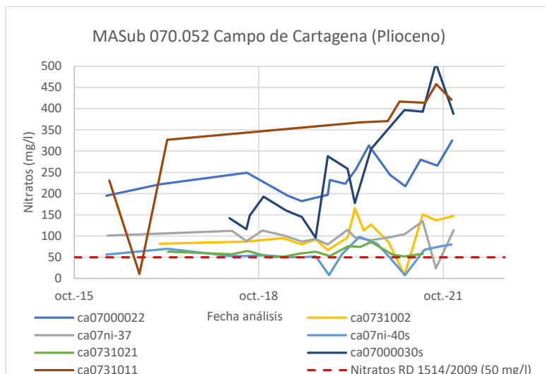
Figura 37 Evolución en las estaciones de muestreo que presentan incumplimiento por concentraciones de nitratos en el año 2020 en la masa de agua subterránea 070.052 Campo de Cartagena (acuífero Cuaternario y Plioceno).
