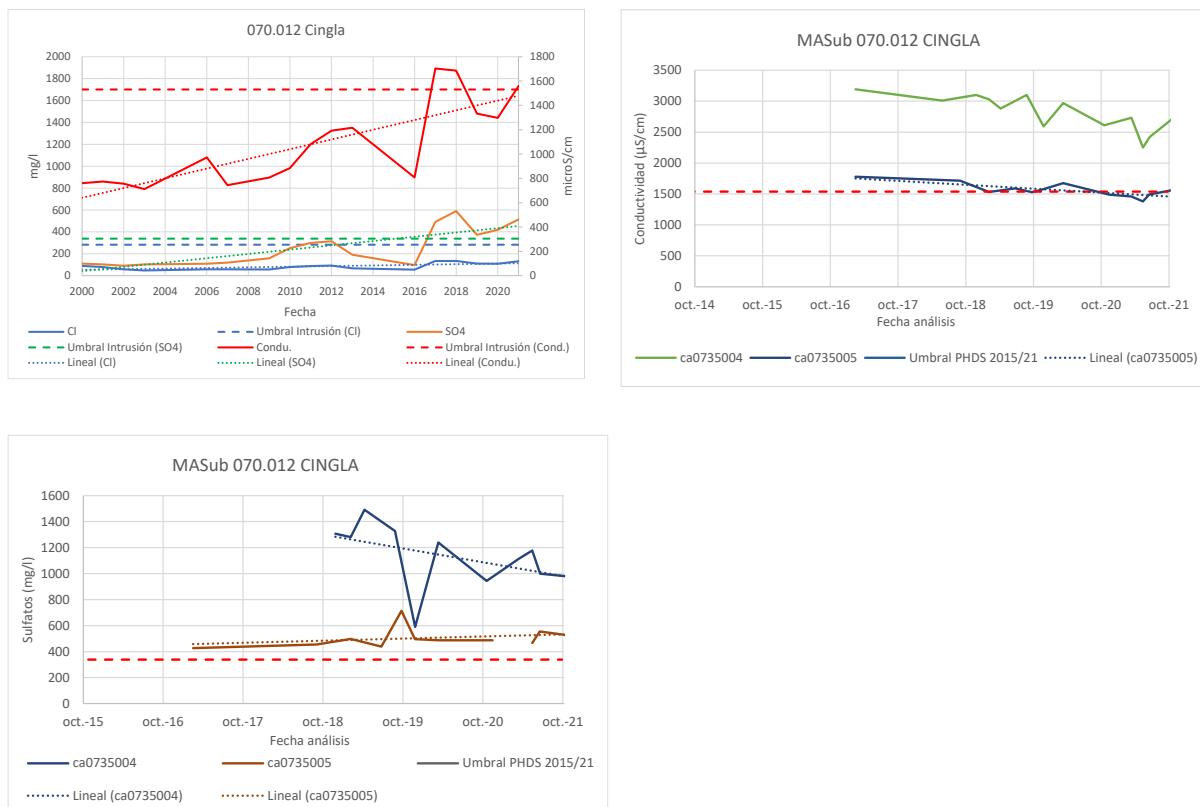
Figura 40 Evolución de puntos de control que presentan incumplimientos por conductividad y sulfatos en el año 2020 en la masa de agua subterránea 070.012 Cingla.
