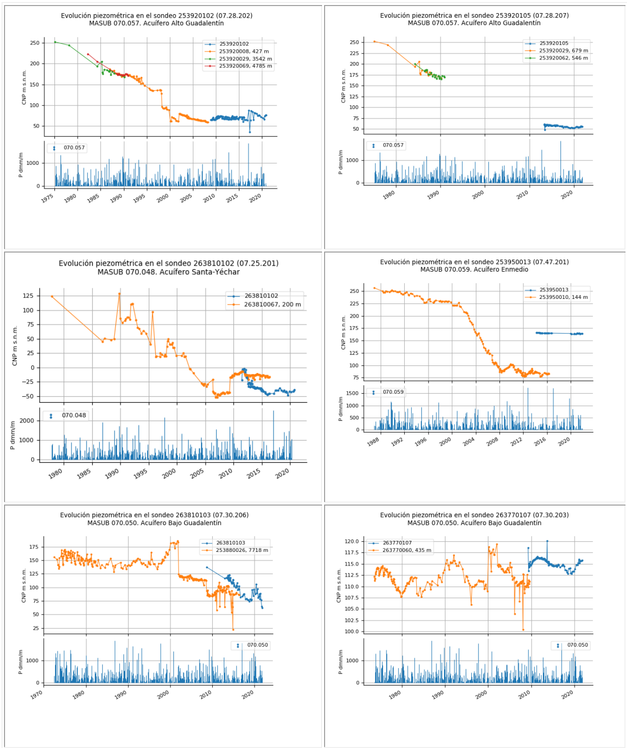
Figura 24 Evolución piezométrica en MASub donde se detecta una interrupción del deterioro temporal
