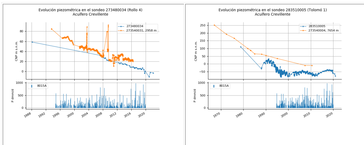
Figura 23 Evolución piezométrica en acuíferos de las MASub 070.031 Sierra de Crevillente (Fuente: Gráficas de evolución piezométrica en puntos de control de la DPA).
