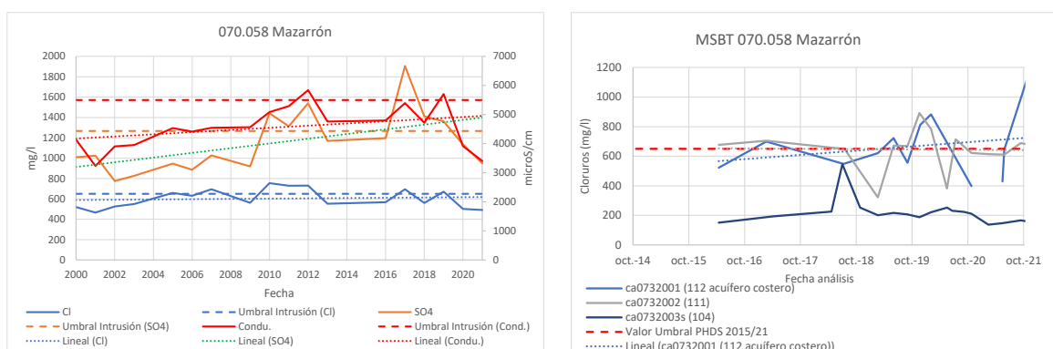
Figura 42 Evolución de la concentración media de cloruros, conductividad y sulfatos y evolución de los incumplimientos de cloruros en la MASUB 070.058 Mazarrón.
