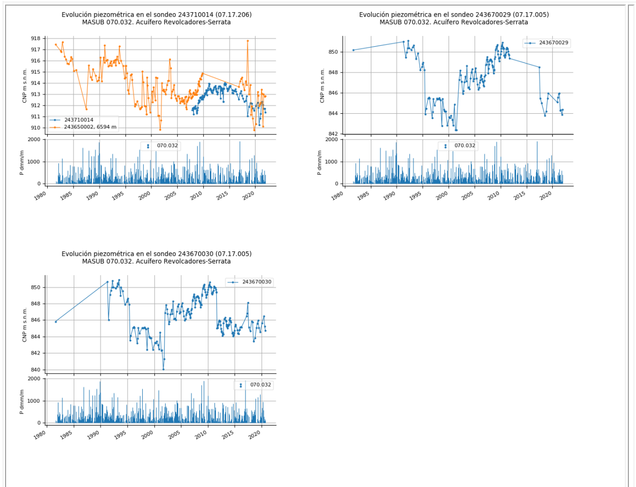
Figura 15 Evolución piezométrica en el acuífero Revolcadores-Serrata. MASub 070.032.
