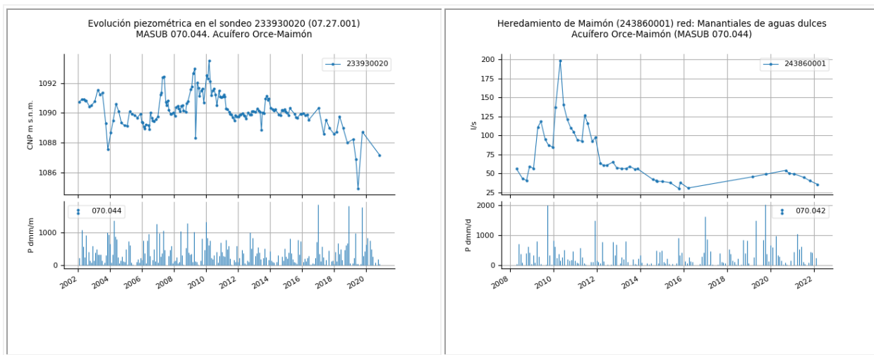
Figura 16 Evolución piezométrica en el acuífero compartido Orce-Maimón. MASub 070.044 Vélez Blanco-María.
