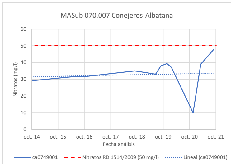
Figura 45 Evolución de la estación de muestreo representativa de la masa de agua subterránea 070.007 Conejeros-Albatana.
