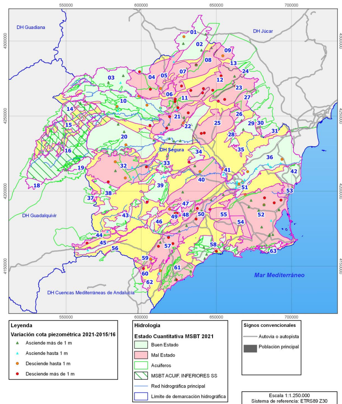
Figura 33 Evolución piezométrica media en el periodo 2015-2021.
