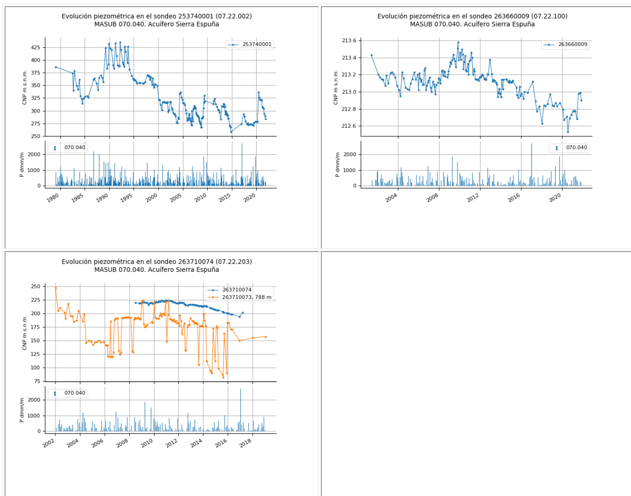
Figura 25 Evolución piezométrica en el acuífero Sierra Espuña-Mula-MASub 070.040-
