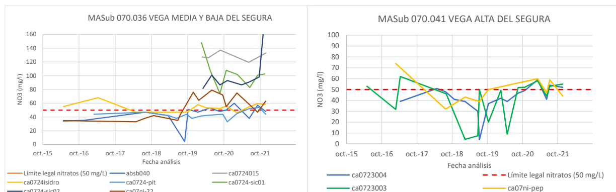
Figura 34 Evolución de concentraciones de nitratos en las MASub 070.036 Vega Media y Baja del Segura y 070.041 Vega Alta del Segura
