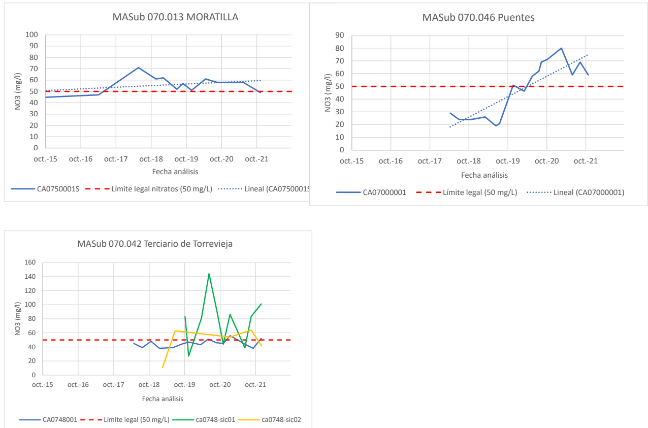
Figura 35 Evolución de puntos de control que presentan incumplimiento por concentraciones de nitratos en el año 2020 en las masas de agua subterránea 070.013 Moratillas, 070.042 Terciario de Torrevieja y 070.046 Puentes.
