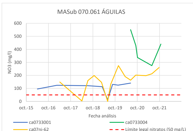
Figura 36 Evolución en las estaciones de muestreo que presentan incumplimiento por concentraciones de nitratos en la masa de agua subterránea 070.061 Águilas
