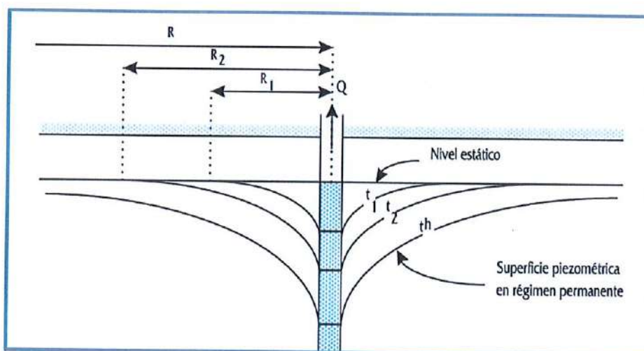
Esquema 2 Evolución del cono de descensos en un pozo de bombeo a lo largo del tiempo ( t_1 , t_2 ...) y del radio de influencia ( R_1 , R_2 ...). Fuente: Universidad Politécnica de Cataluña. https://www.upc.edu/ca
