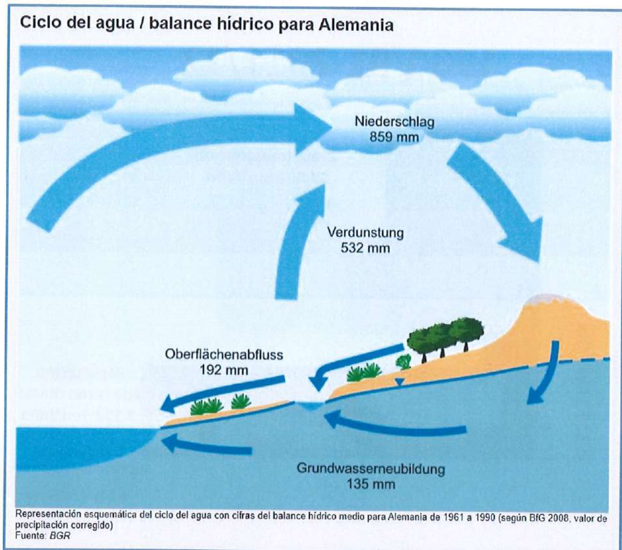
Figura 3 En el esquema del ciclo natural del agua en Alemania igualmente vemos como la P menos la ETR es la suma de la E más la R . 859 - 532 = 192 + 135 .
