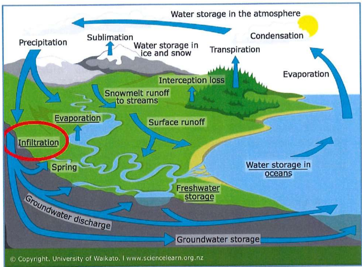
Figura 11 El ciclo del agua de la Universidad de Waikato, Nueva Zelanda. Hemos resaltado con un círculo rojo el concepto de "Infiltration" (infiltración) que como vemos es la suma del flujo fluvial y del flujo subterráneo directo al mar (Groundwater discharge) y que alimenta los almacenamientos subterráneos (Groundwater storage)
