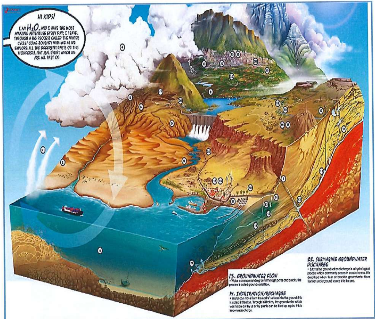
Figura 4 Otra imagen conceptual que hemos simplificado para su mejor comprensión del ciclo del agua en Alemania del BGR (Instituto Federal de Geociencias y Recursos Naturales). Destacamos que el concepto "Infiltración/Recarga" (14) está ligado al flujo de agua subterránea al mar (22) procedente del continente (13)
