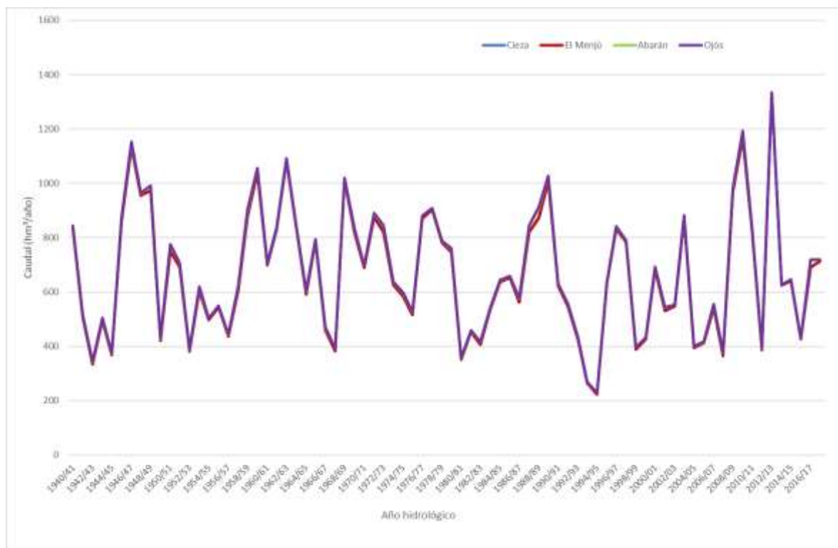
Figura 20. Caudal medio (hm³/año) en el Río Segura hasta Ojós
