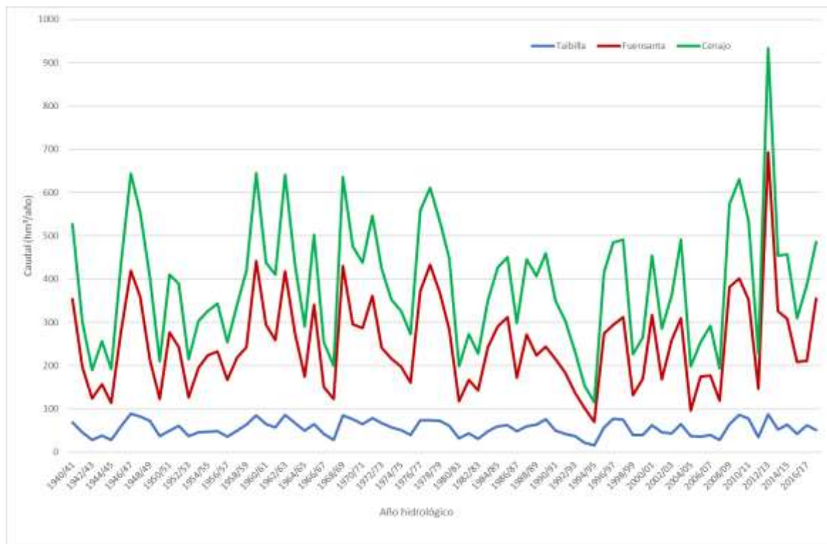
Figura 16. Caudal medio ( \text{hm}^3/\text{año} ) en el Alto Segura
