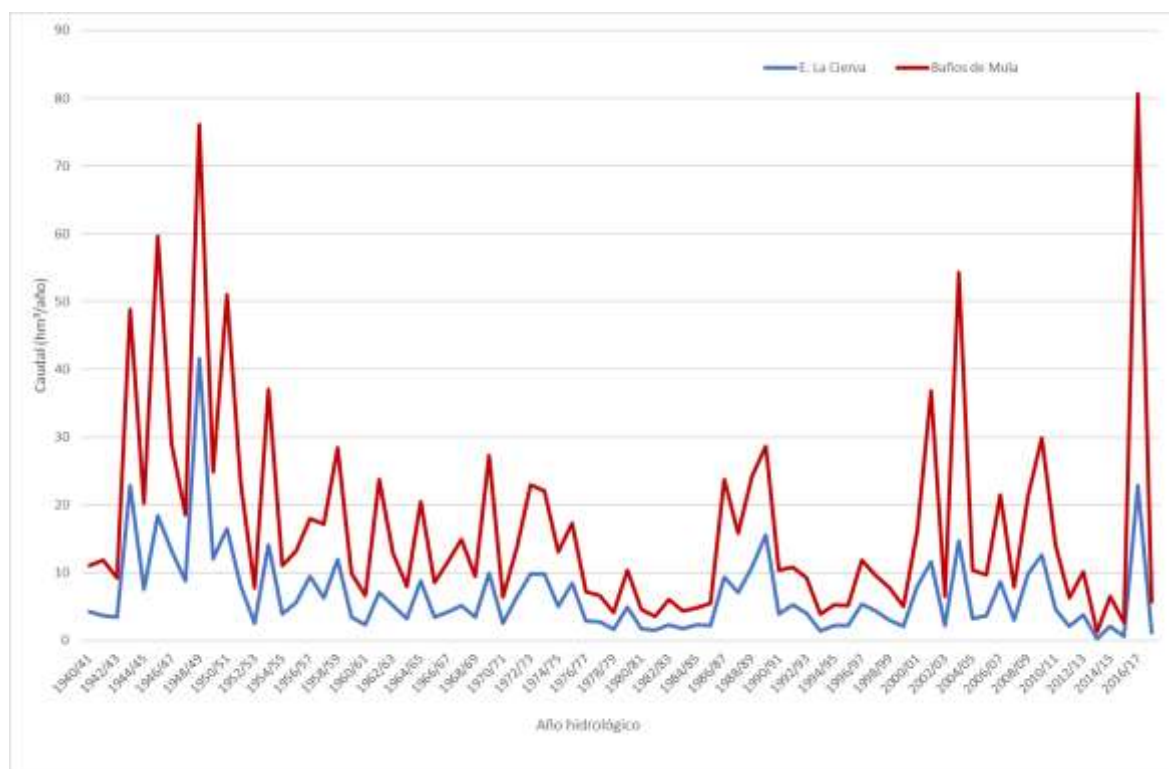
Figura 18. Caudal medio (hm³/año) en el Río Mula
