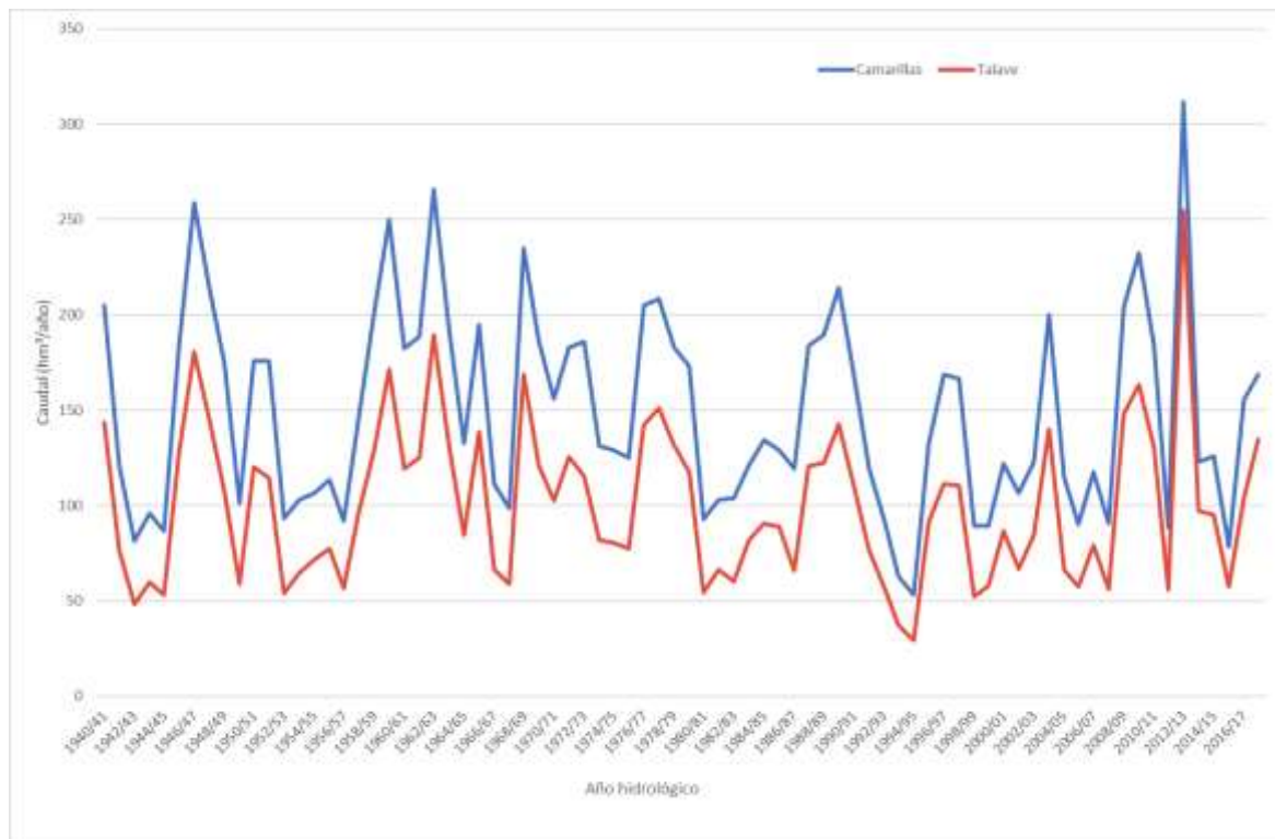
Figura 15. Caudal medio ( \text{hm}^3/\text{año} ) en el Río Mundo
