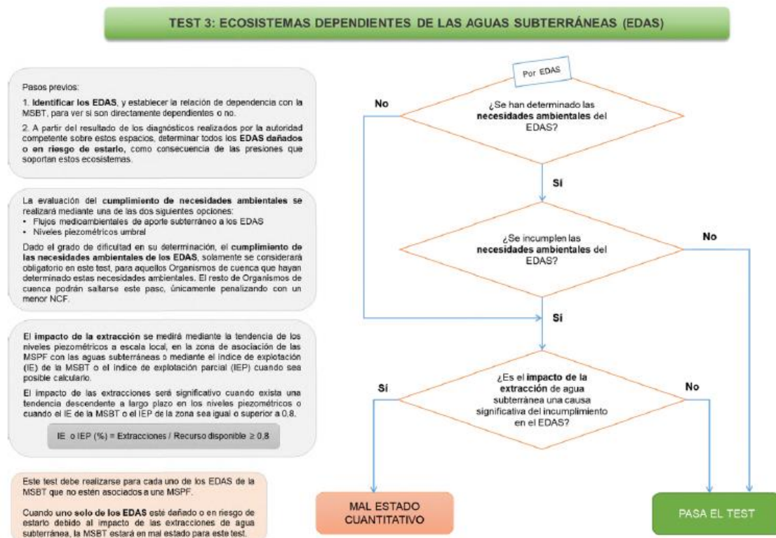
Figura 10. Esquema del test 3 de EDAS de la evaluación del estado cuantitativo en MSBT (MITERD, 2020)
