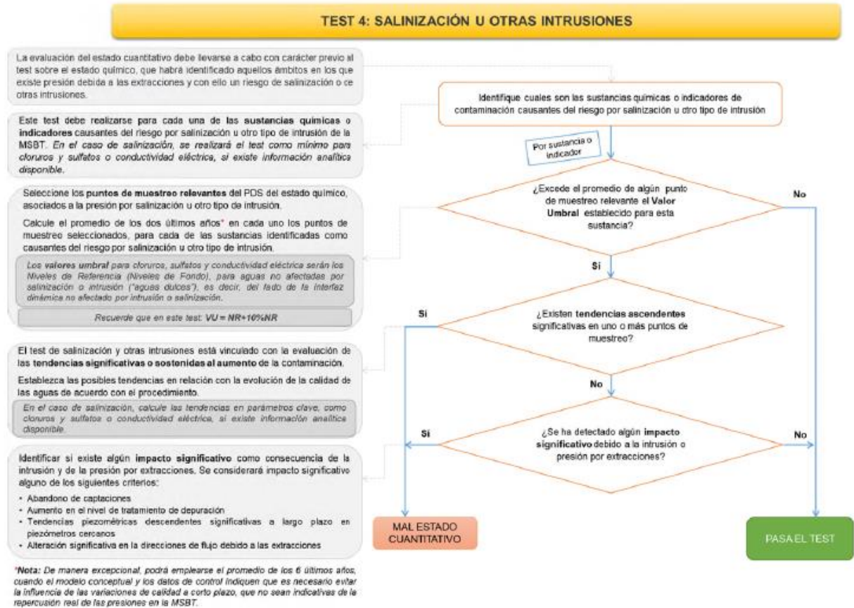
Figura 18. Esquema del test 4 de salinización de evaluación del estado cuantitativo en MSBT (MITERD,2020)
