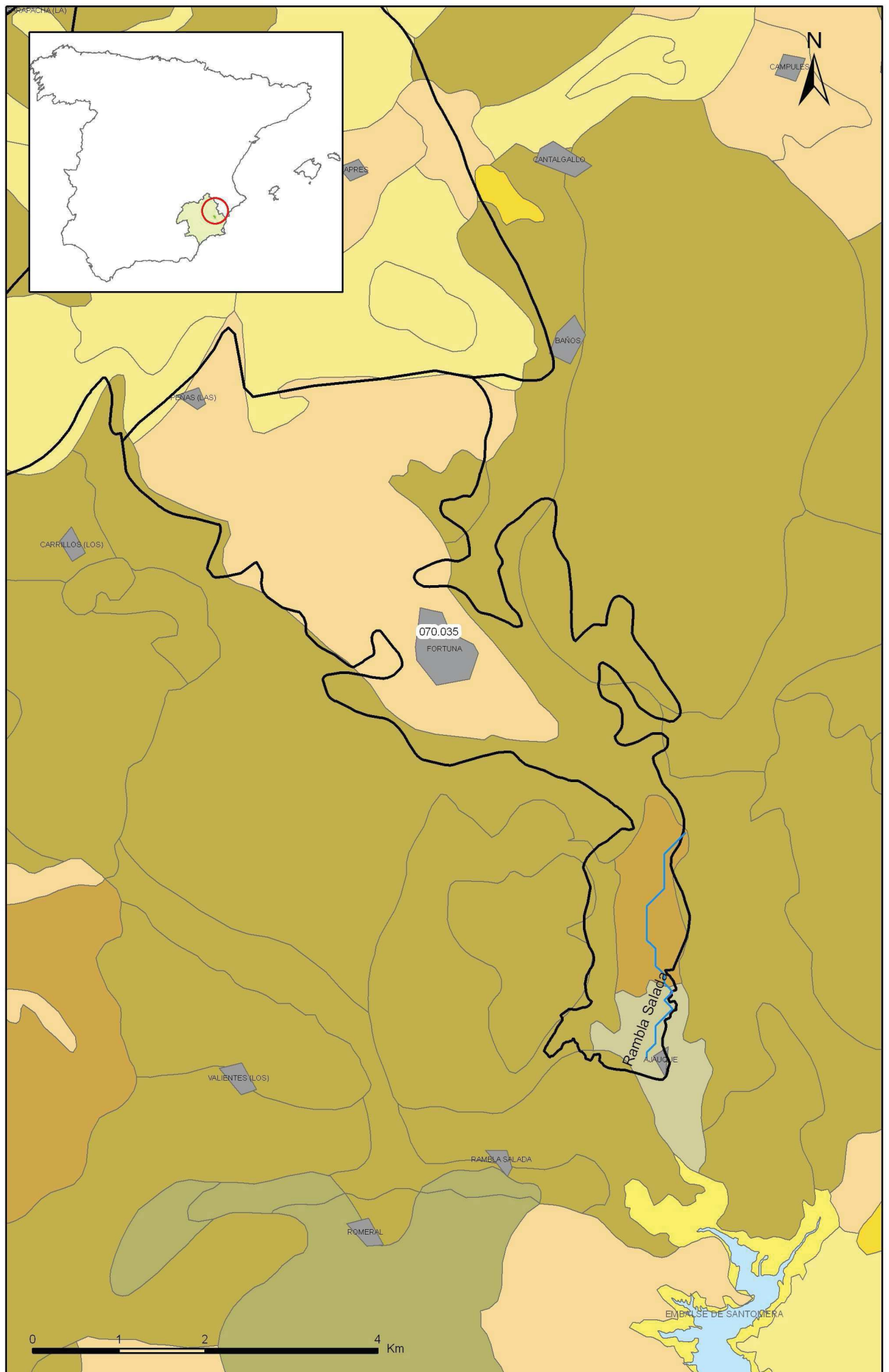
Mapa 4.1 Mapa de suelos de la masa Cuaternario de Fortuna (070.035)
