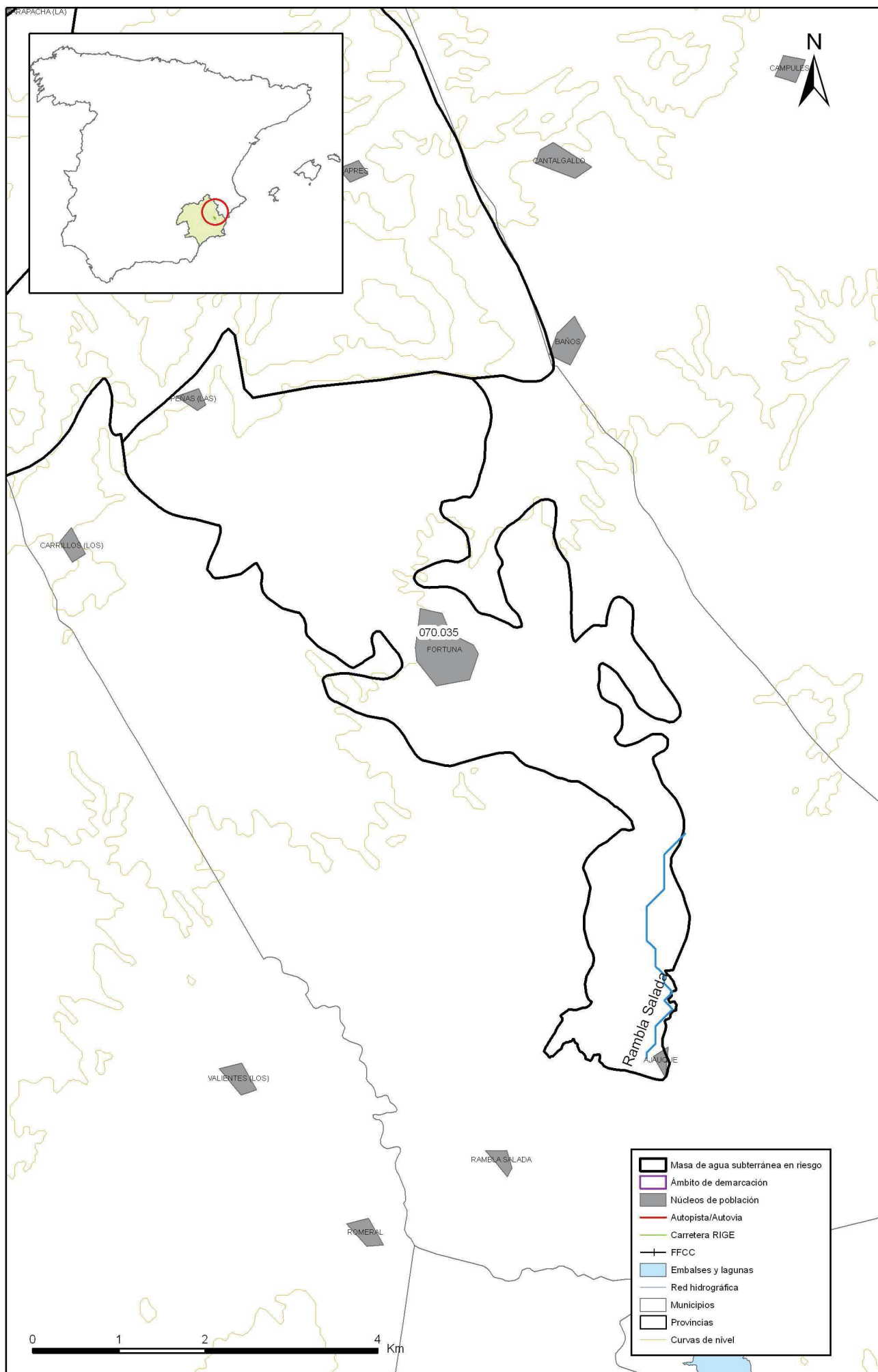
Mapa 1.1 Mapa base cartográfica de la masa Cuaternario de Fortuna (070.035)
