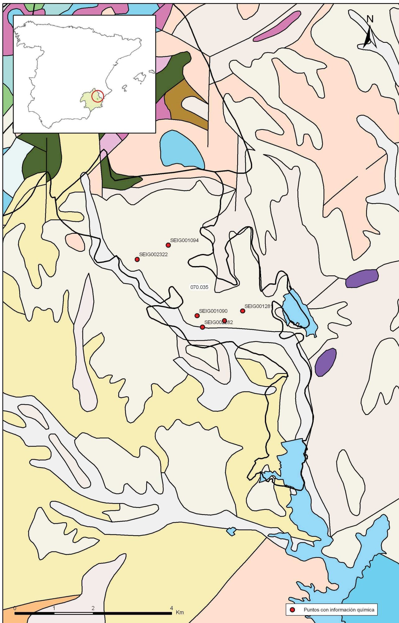
Mapa 10.1 Mapa de situación de puntos en la determinación de niveles de referencia de la masa Cuaternario de Fortuna (070.035)
