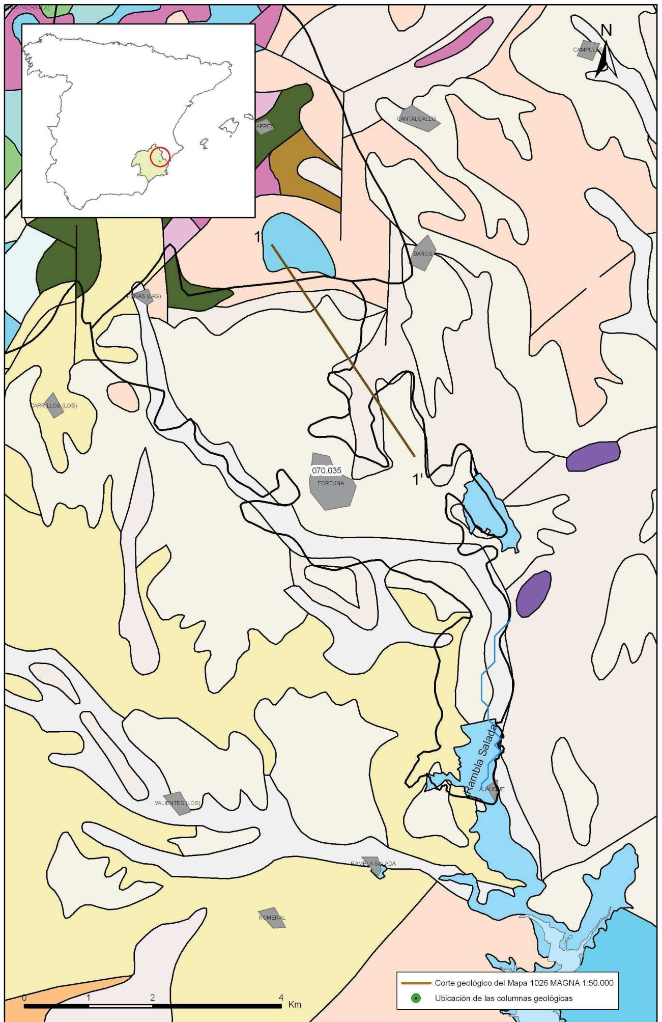
Mapa 2.1 Mapa geológico de la masa Cuaternario de Fortuna (070.035)
