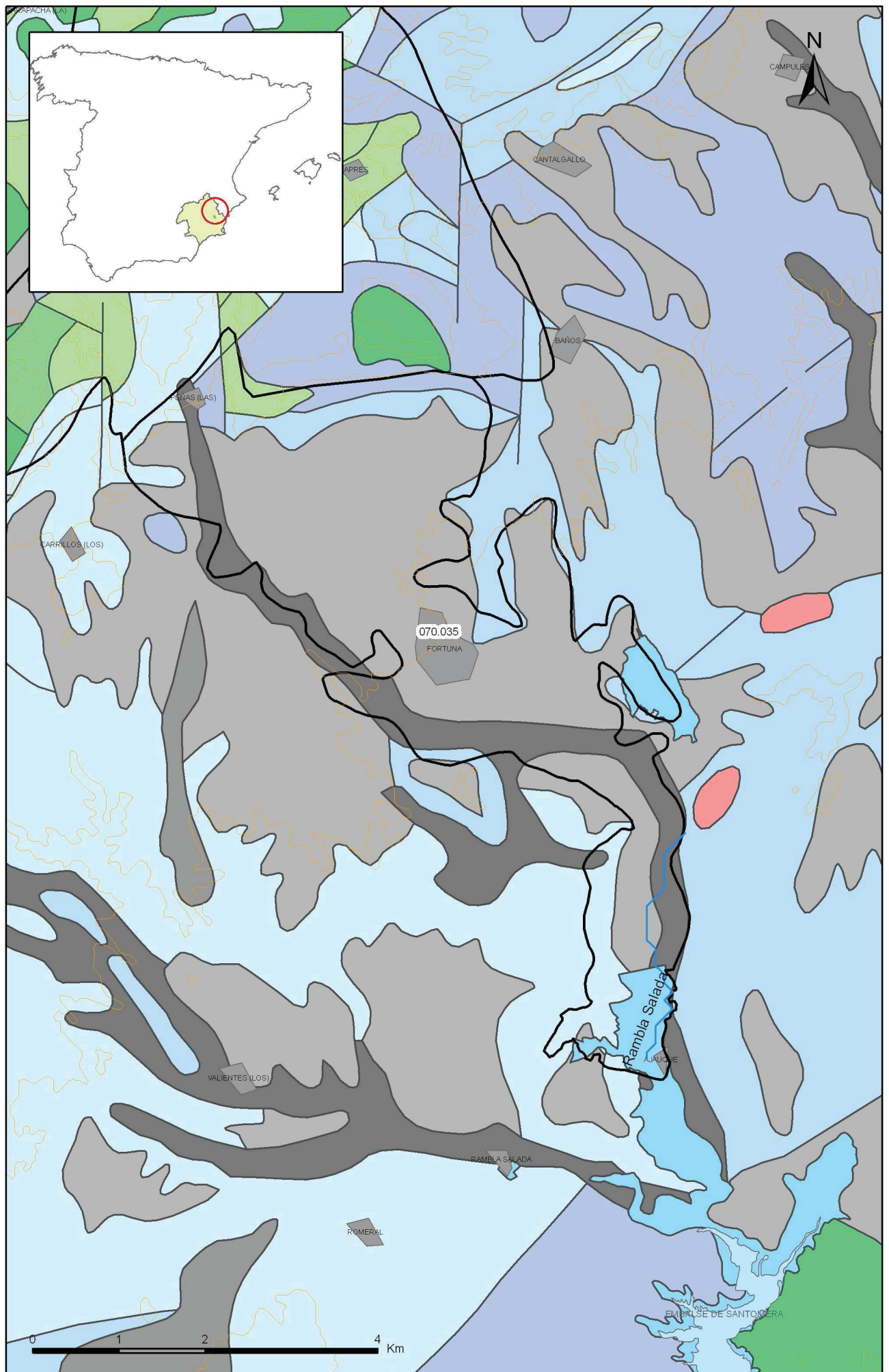
Mapa 3.1 Mapa de permeabilidades según litología de la masa Cuaternario de Fortuna (070.035)
