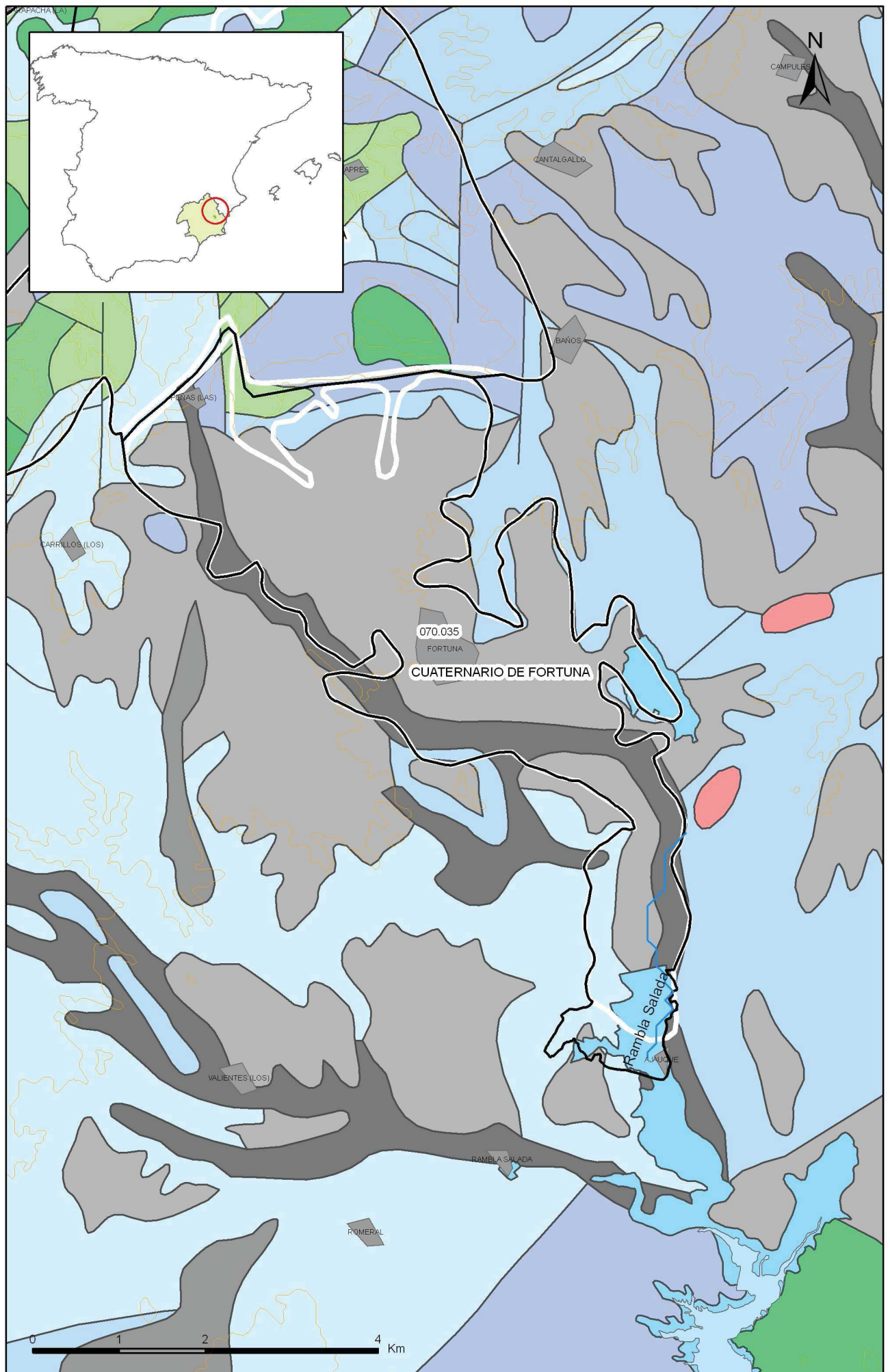
Mapa 3.2 Mapa hidrogeológico con especificación de acuíferos de la masa Cuaternario de Fortuna (070.035)
