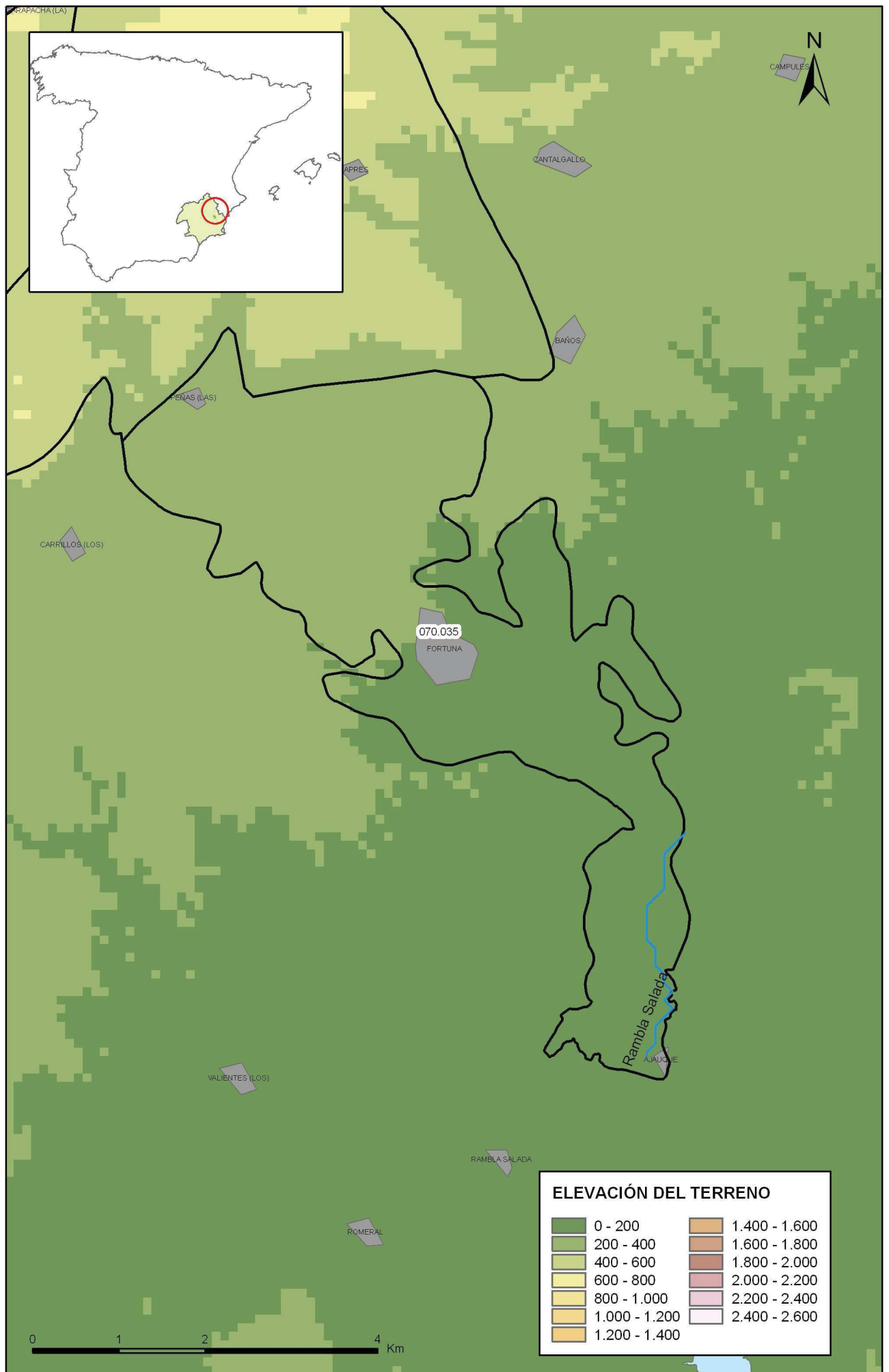
Mapa 1.2 Mapa digital de elevaciones de la masa Cuaternario de Fortuna (070.035)
