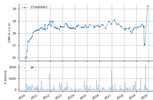
Evolución de la cota piezométrica en el sondeo 273680063 MASub 070.036. Acuífero Vegas Media y Baja del Segura
