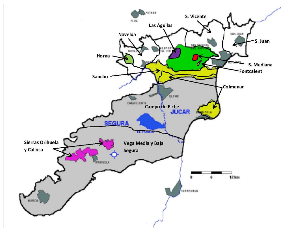
Figura 3.1. Acuíferos de la MASub Vega Media y Baja del Segura y MASub Bajo Vinalopó (Fuente: IGME-DGA, 2020)
