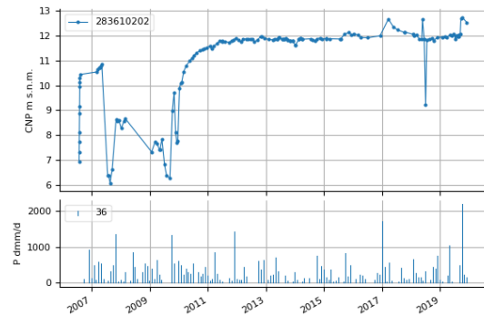
Evolución de la cota piezométrica en el sondeo 283610202 MASub 070.036. Acuífero Vegas Media y Baja del Segura
