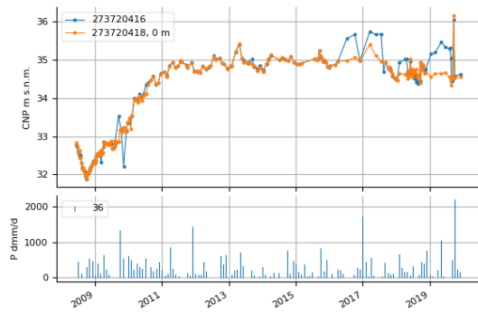
Evolución de la cota piezométrica en el sondeo 273720416 MASub 070.036. Acuífero Vegas Media y Baja del Segura
