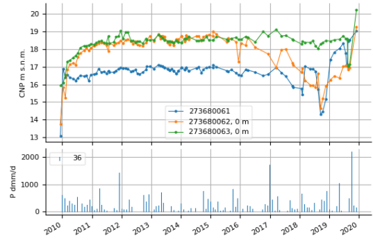
Evolución de la cota piezométrica en el sondeo 273680061 MASub 070.036. Acuífero Vegas Media y Baja del Segura
