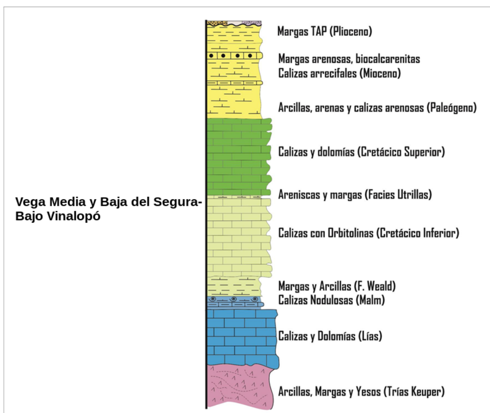
Figura 2.2. Columna litoestratigráfica simplificada del dominio Prebético de la MASub Vega Media y Baja del Segura (tercio septentrional)
