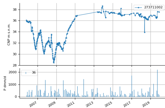
Evolución de la cota piezométrica en el sondeo 273711002 MASub 070.036. Acuífero Vegas Media y Baja del Segura
