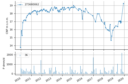
Evolución de la cota piezométrica en el sondeo 273680062 MASub 070.036. Acuífero Vegas Media y Baja del Segura
