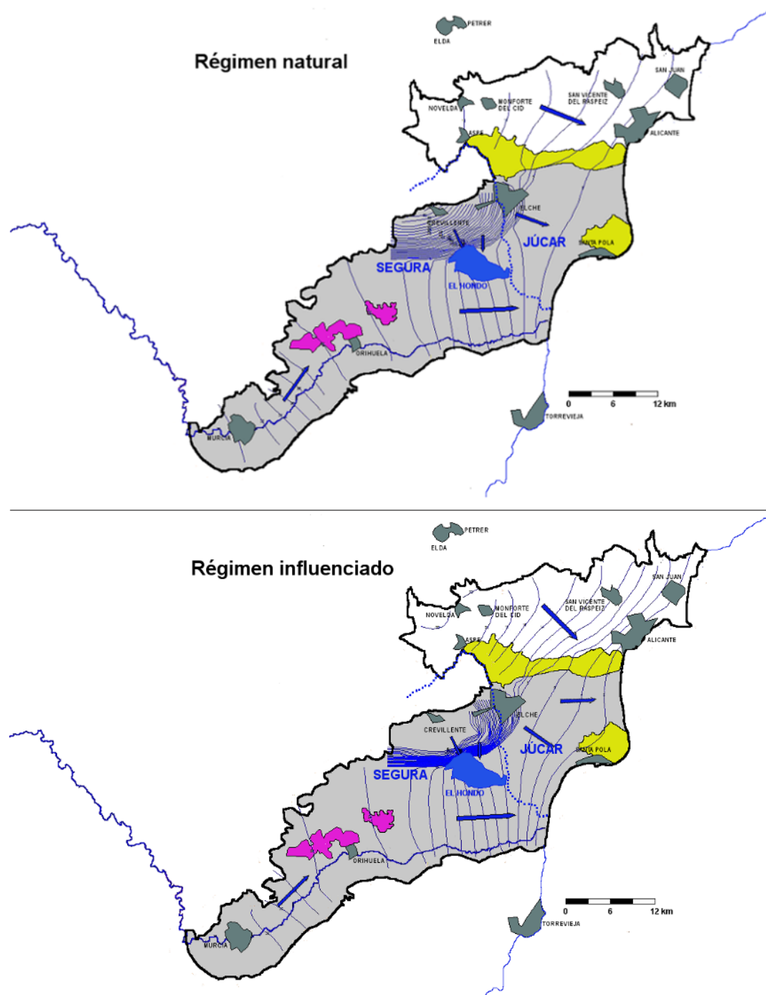
Figura 3.5. MASub Vega Media y Baja del Segura-Bajo Vinalopó. Superficie piezométrica deducida en régimen natural y en régimen influenciado (alterado por bombeos) al final del año 2017
