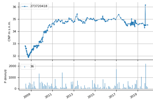
Evolución de la cota piezométrica en el sondeo 273720418 MASub 070.036. Acuífero Vegas Media y Baja del Segura
