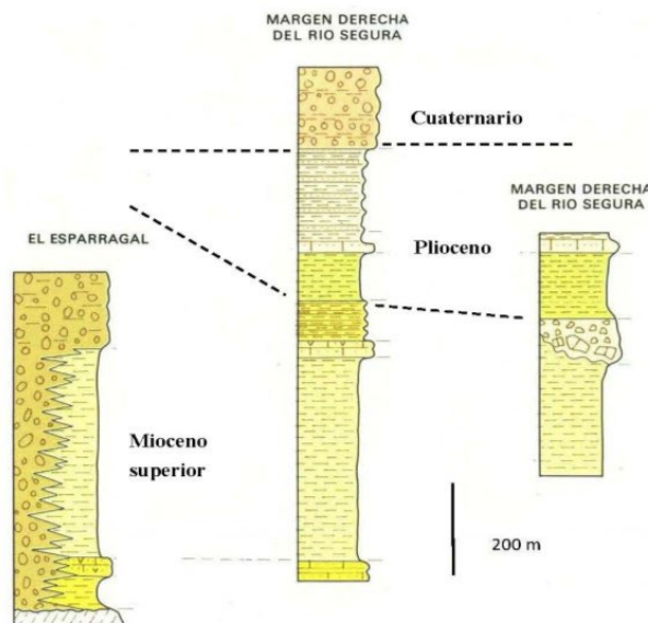
Figura 2.4. Serie litoestratigráfica del Terciario-Cuaternario de la MASub Vega Media y Baja del Segura (fosas tectónicas). MAGNA Hoja 27-36 Orihuela (IGME, 1972)
