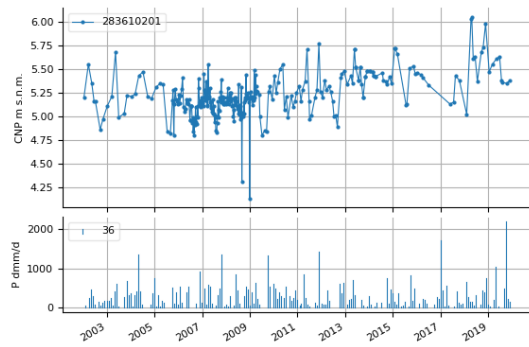
Evolución de la cota piezométrica en el sondeo 283610201 MASub 070.036. Acuífero Vegas Media y Baja del Segura
