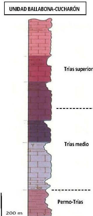
Figura 2.3. Columna litoestratigráfica simplificada del dominio de las Zonas Internas de la MASub Vega Media y Baja del Segura (sector meridional). MAGNA Hoja 27-36 Orihuela (IGME, 1972)
