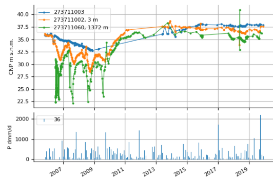
Evolución de la cota piezométrica en el sondeo 273711003 MASub 070.036. Acuífero Vegas Media y Baja del Segura
