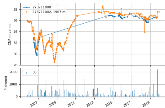
Evolución de la cota piezométrica en el sondeo 273711080 MASub 070.036. Acuífero Vegas Media y Baja del Segura
