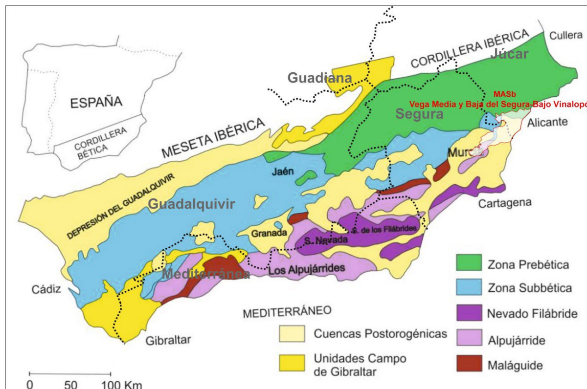
Figura 2.1 La MASub Vega Media y Baja del Segura en el marco de las Cordilleras Béticas (Mod. Fernandez y Gil 1989)
