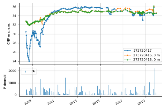
Evolución de la cota piezométrica en el sondeo 273720417 MASub 070.036. Acuífero Vegas Media y Baja del Segura
