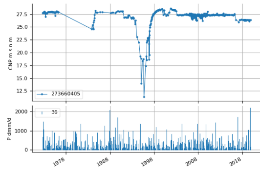
Evolución de la cota piezométrica en el sondeo 273660405 MASub 070.036. Acuífero Vegas Media y Baja del Segura
