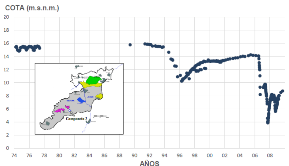
Figura 3.3. Evolución piezométrica en el pozo Campaneta 2. (Fuente: IGME-DGA, 2020)
