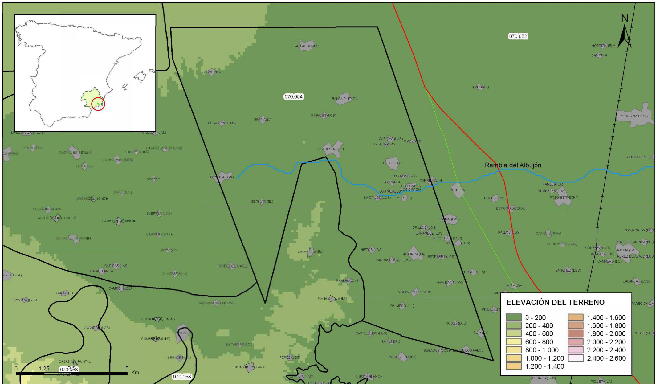
Mapa 1.2 Mapa digital de elevaciones de la masa Triásico de Los Victorias (070.054)
