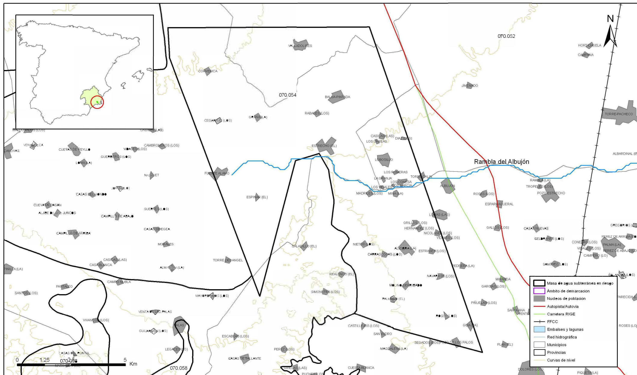
Mapa 1.1 Mapa base cartográfica de la masa Triásico de Los Victorias (070.054)
