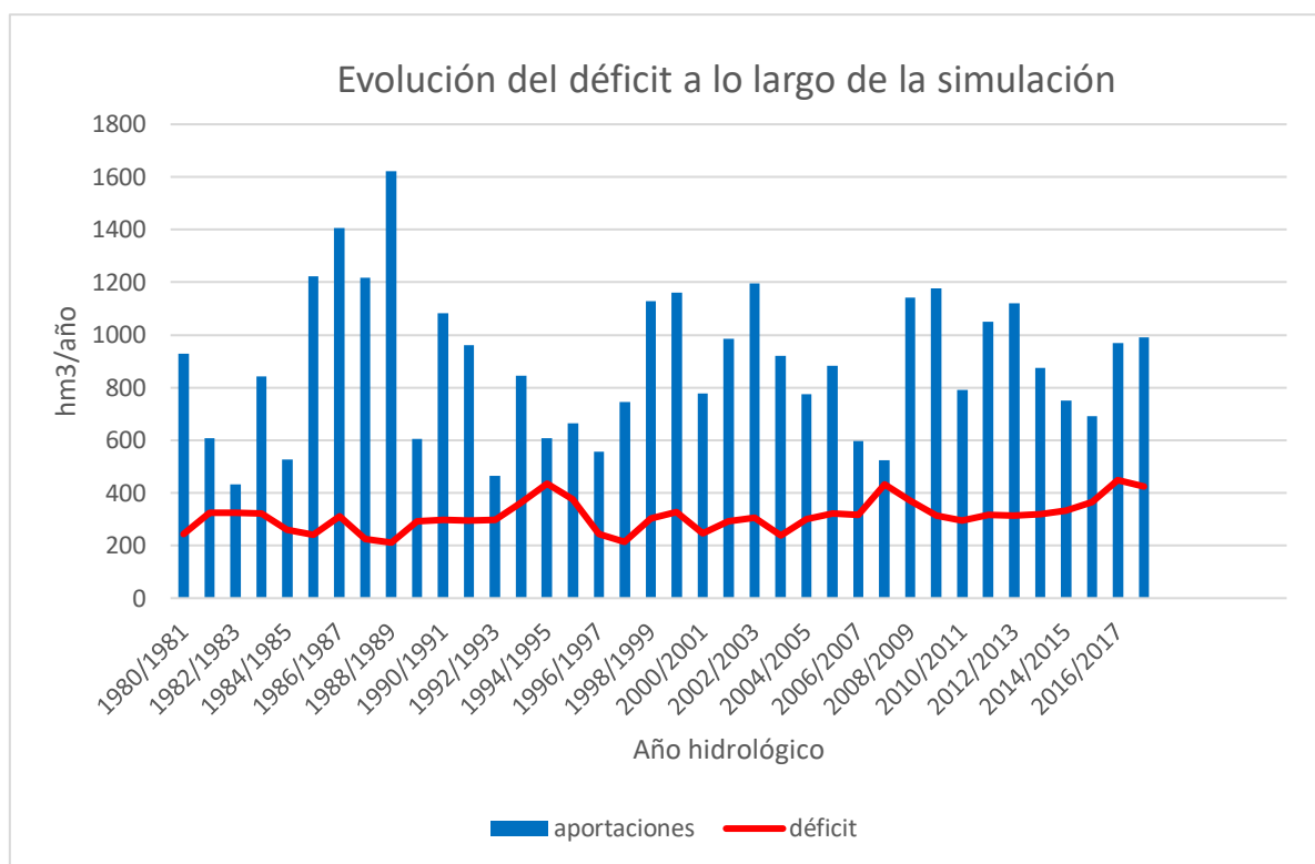
Figura 3. Evolución del déficit a lo largo de la simulación. Horizonte 2021. Periodo 1980/81-2017/18. ATS aplicando las vigentes reglas de explotación 1980/81-2017/18, 295 \text{hm}^3/\text{año}
