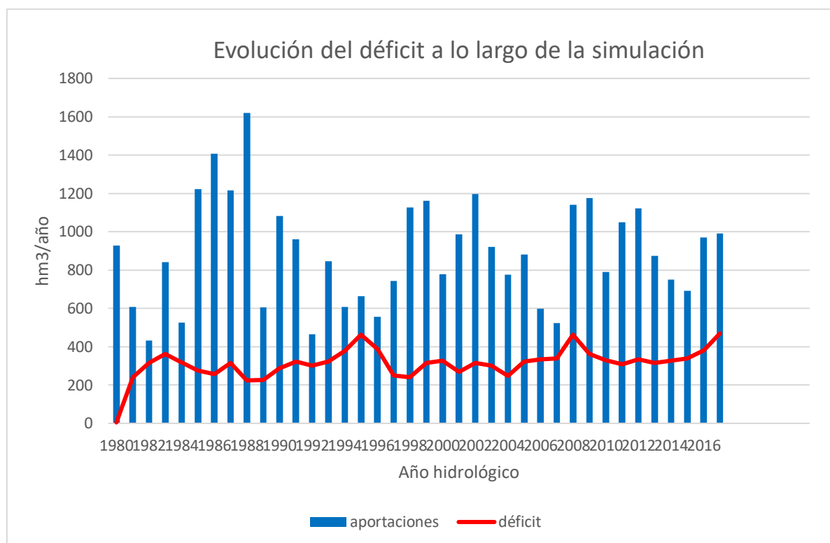
Figura 7. Evolución del déficit a lo largo de la simulación. Horizonte 2039. Periodo 1980/81-2017/18.
