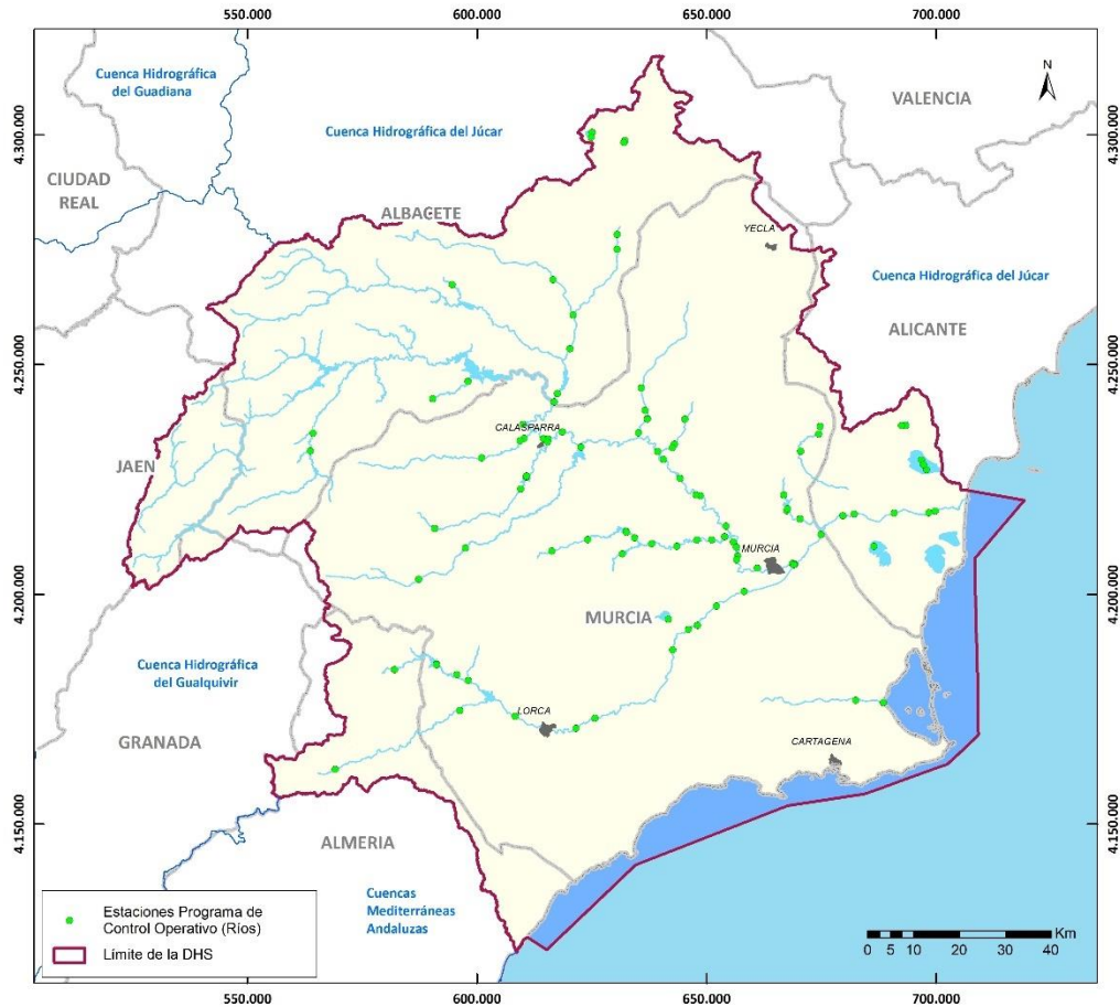
Figura 9. Estaciones del Programa de control operativo de las aguas continentales de la DHS.
