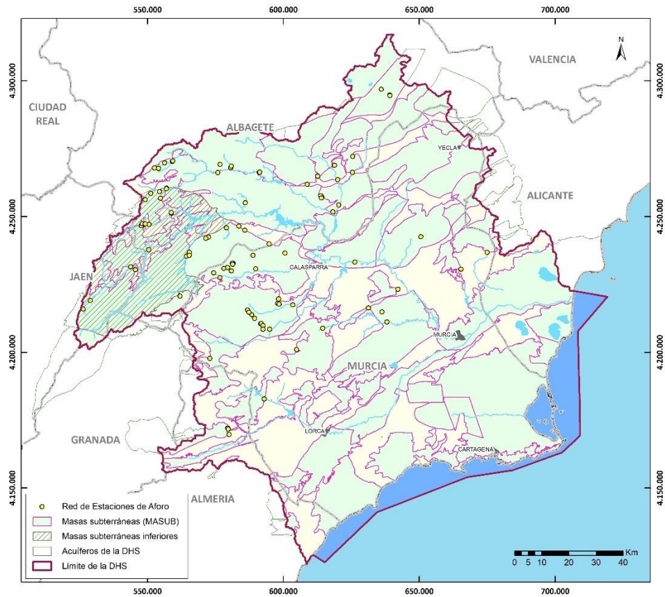
Figura 27. Red foronomía de la DHS, control cuantitativo.
