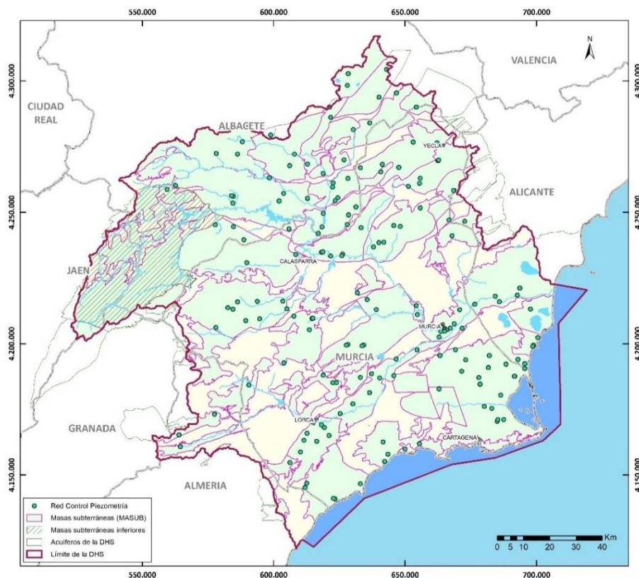
Figura 26. Red piezométrica de la DHS, control cuantitativo.
