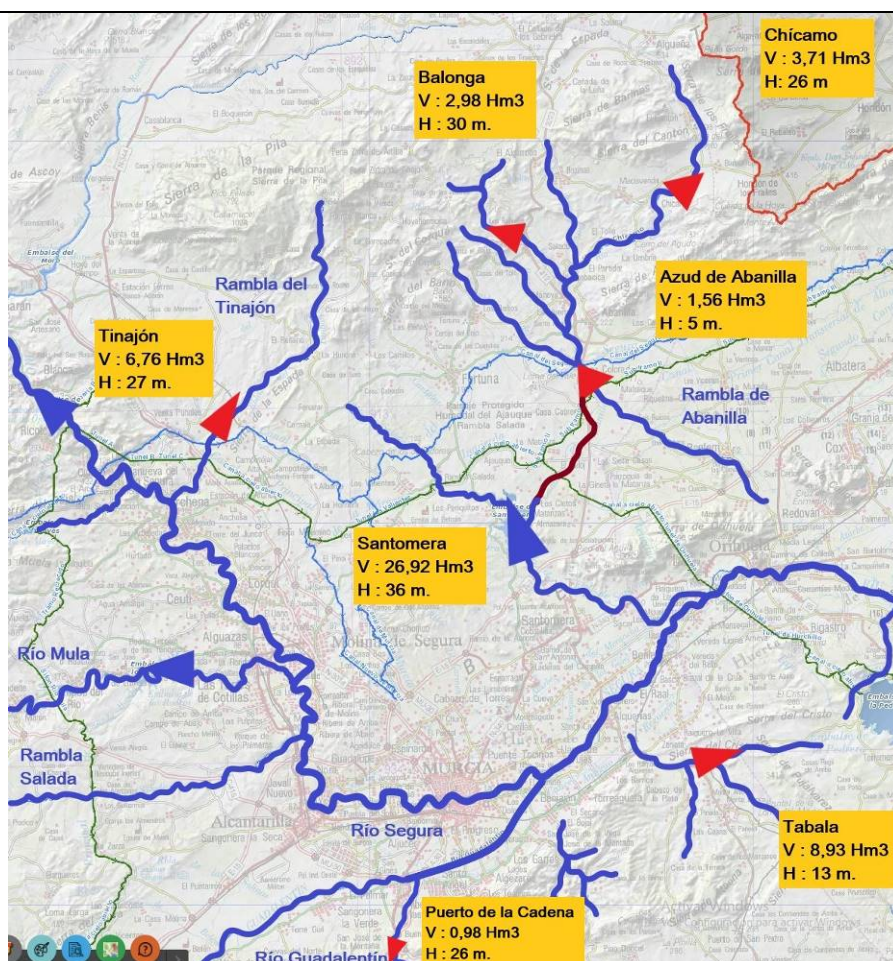
Esquema de actuaciones fuera del llano de inundación propuestas por la Universidad Politécnica de Valencia con el objeto de defender la Vega Baja del Segura frente a inundaciones
