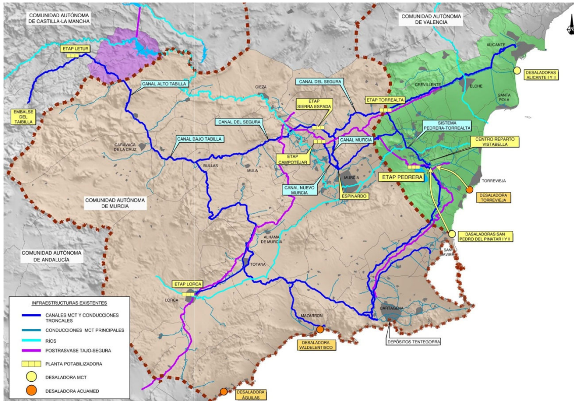
Figura 30. Sistema Hidráulico de la MCT.
