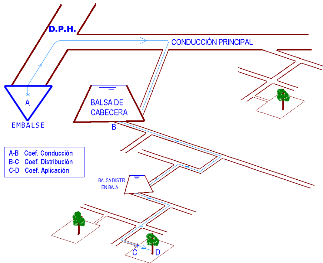
Figura 38. Esquema de regadío modernizado superficial de agua superficial.
