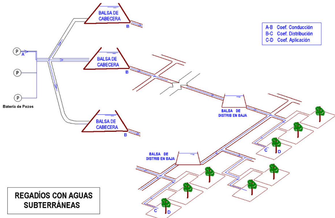
Figura 39. Esquema de regadío de aguas subterráneas.
