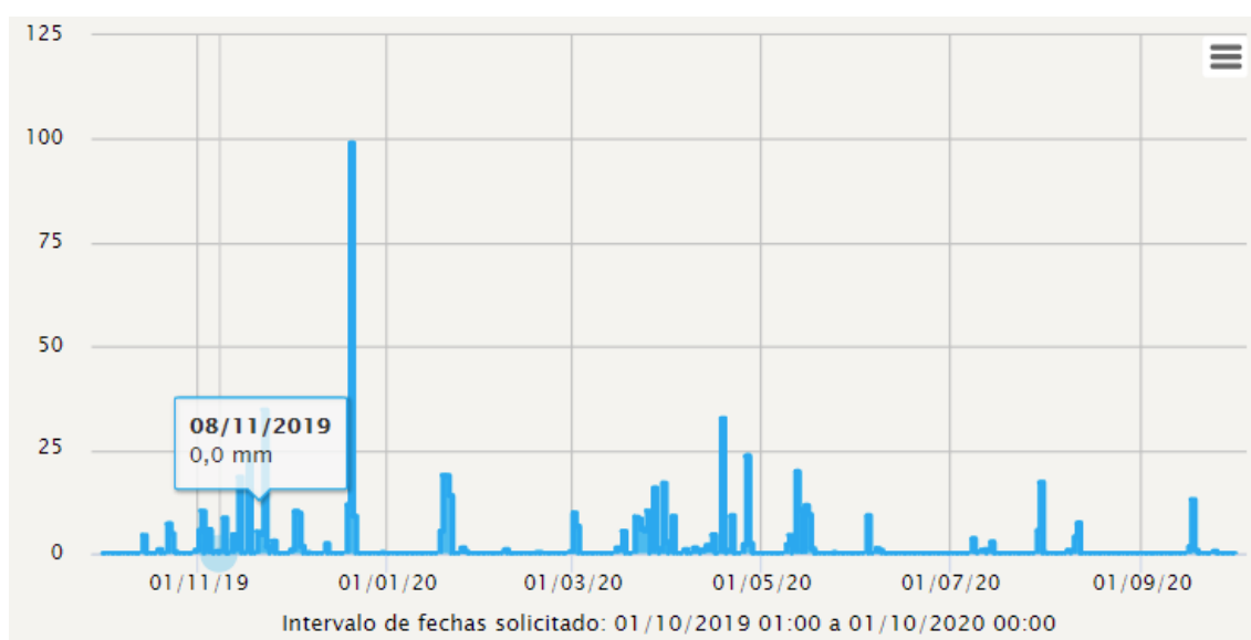
Figura 8. Variación pluviométrica diaria registrada en Las Juntas durante el año hidrológico 2019/20
