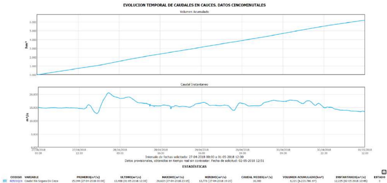
Variación del caudal registrado en la EA de Cieza durante el transcurso del episodio.
