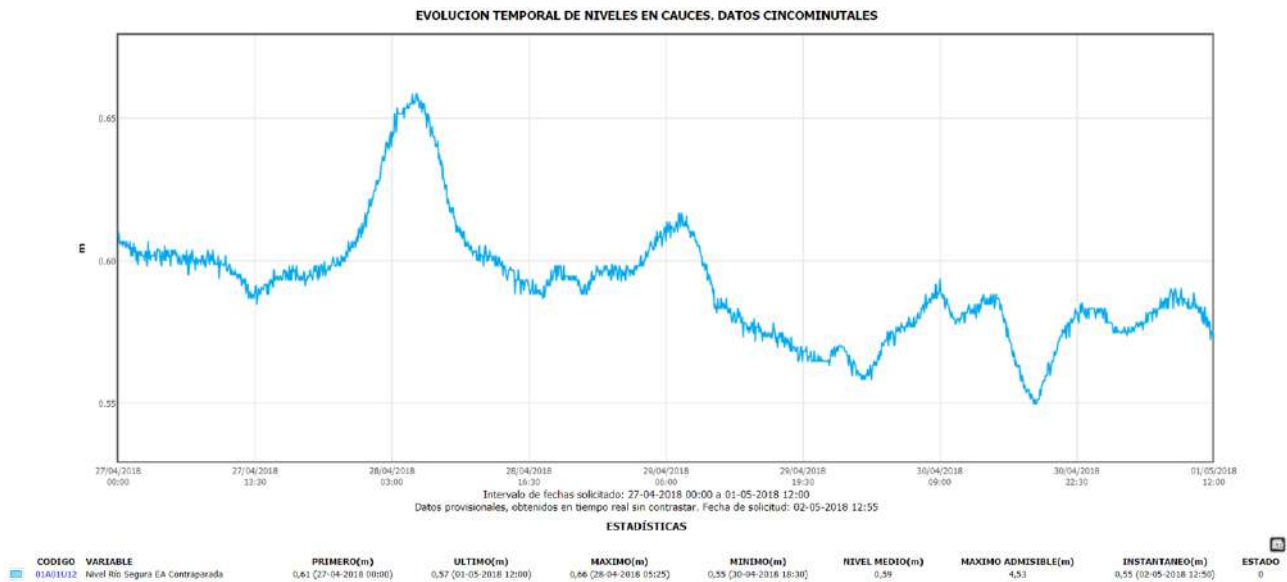
Variación del nivel registrado en la EA de Contraparada durante el transcurso del episodio.
