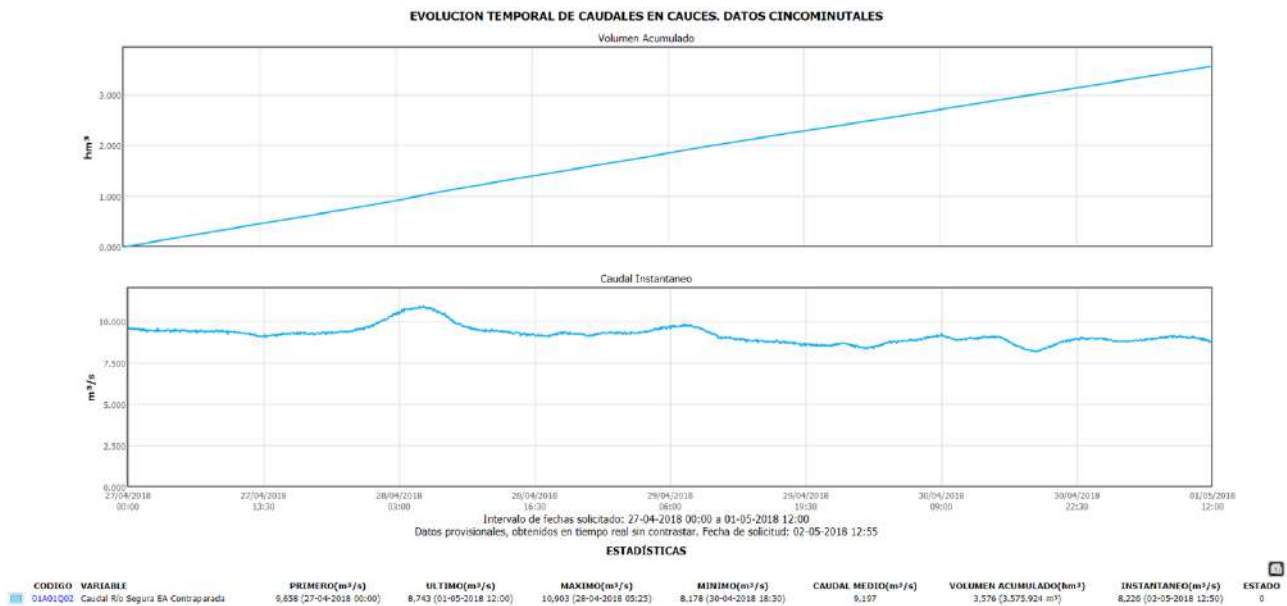
Variación del caudal registrado en la EA de Contraparada durante el transcurso del episodio.
