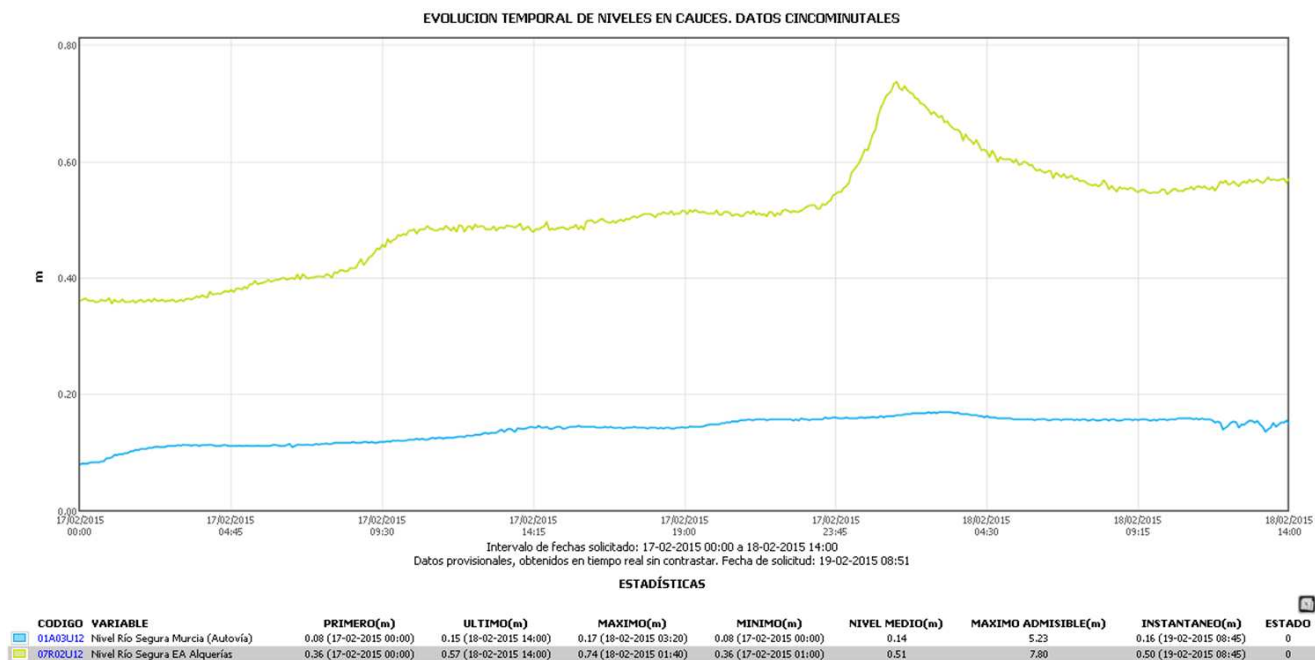
Variación del nivel registrado en Murcia (Autovía) y la EA de Alquerías durante el transcurso del episodio.
