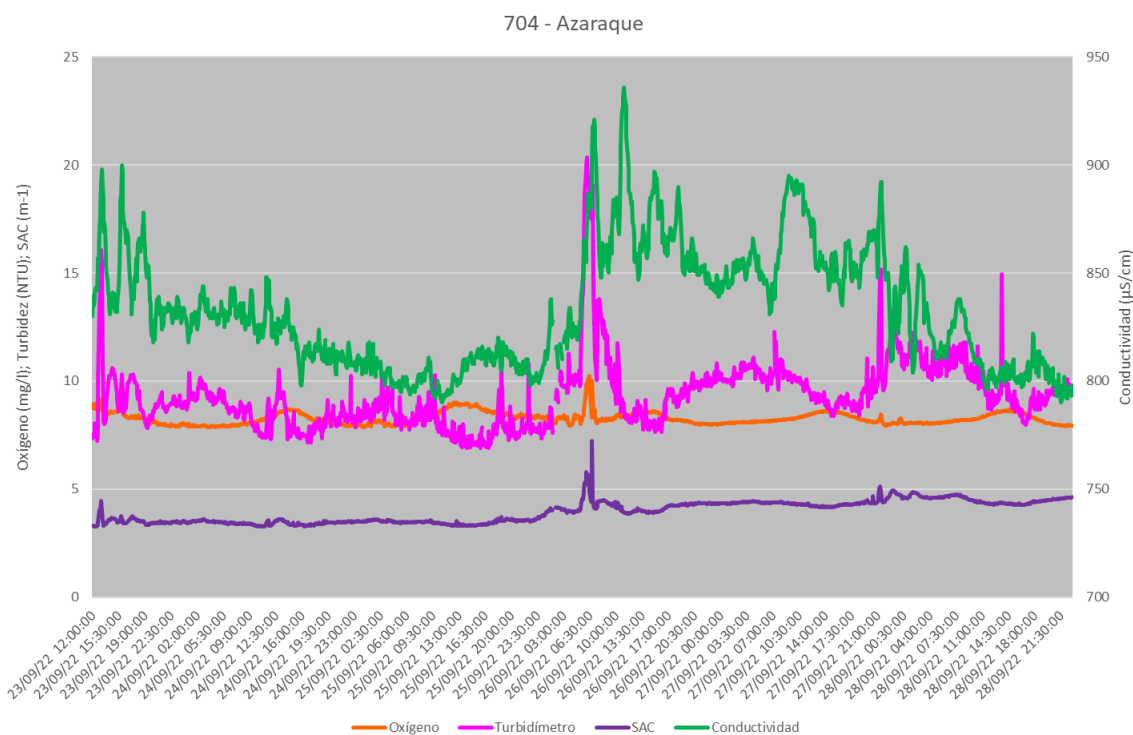
Gráfica 2. Evolución de parámetros en la EA de Azaraque: 23 al 28 de septiembre.
