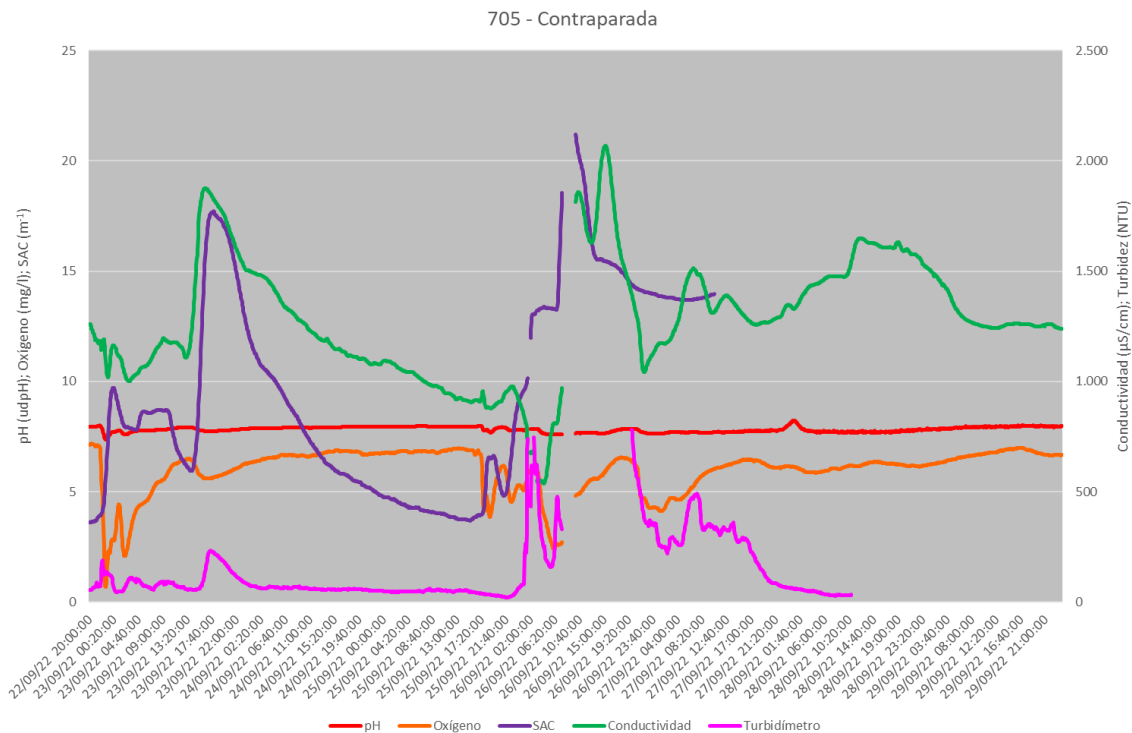
Gráfica 7. Evolución de parámetros en la EA de Contraparada: 22 al 29 de septiembre.
