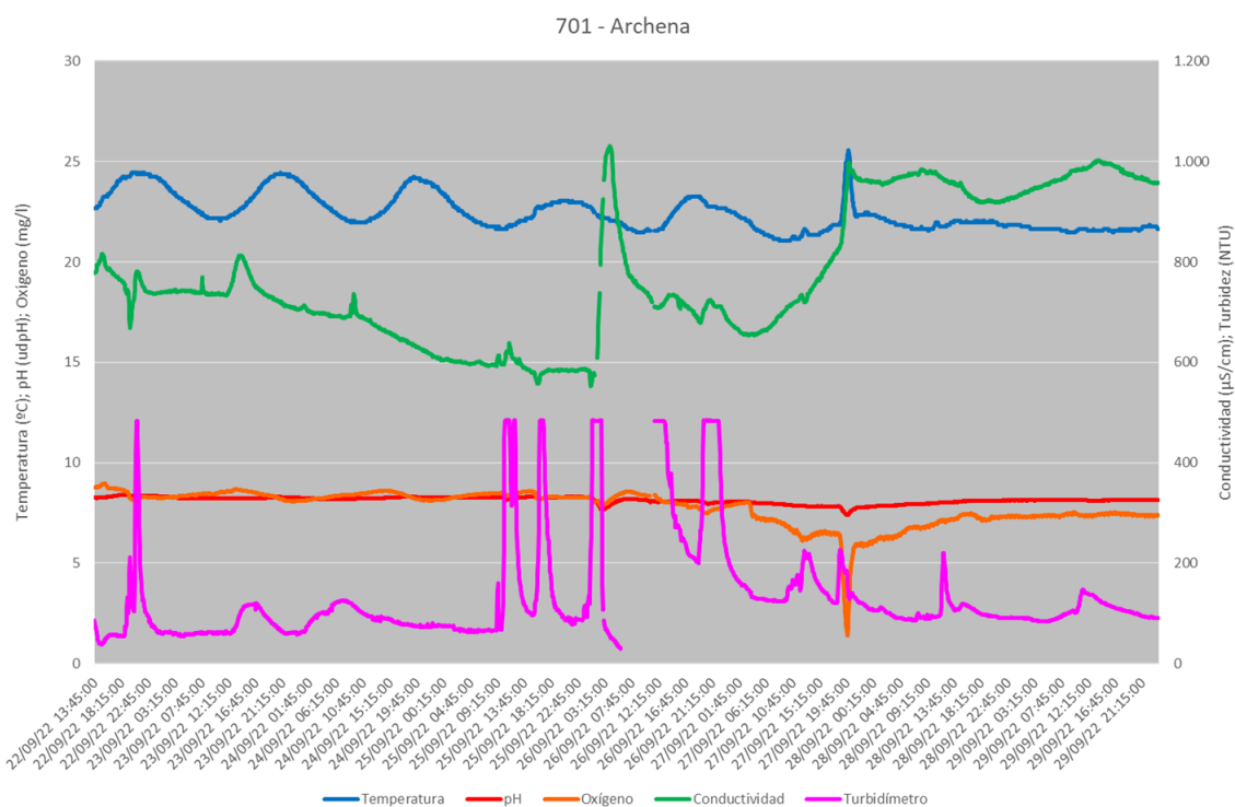
Gráfica 6. Evolución de parámetros en la EA de Archena: 22 al 29 de septiembre.
