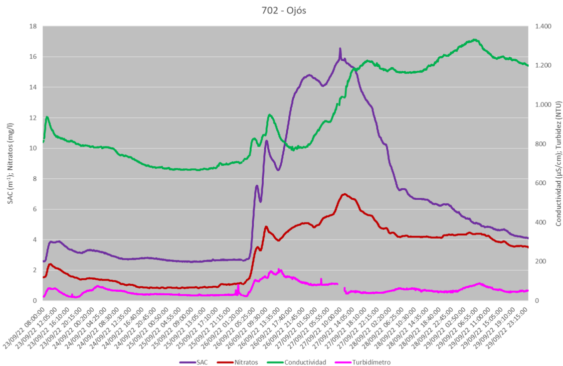
Gráfica 5. Evolución de parámetros en la EA de Ojós: 23 al 29 de septiembre.
