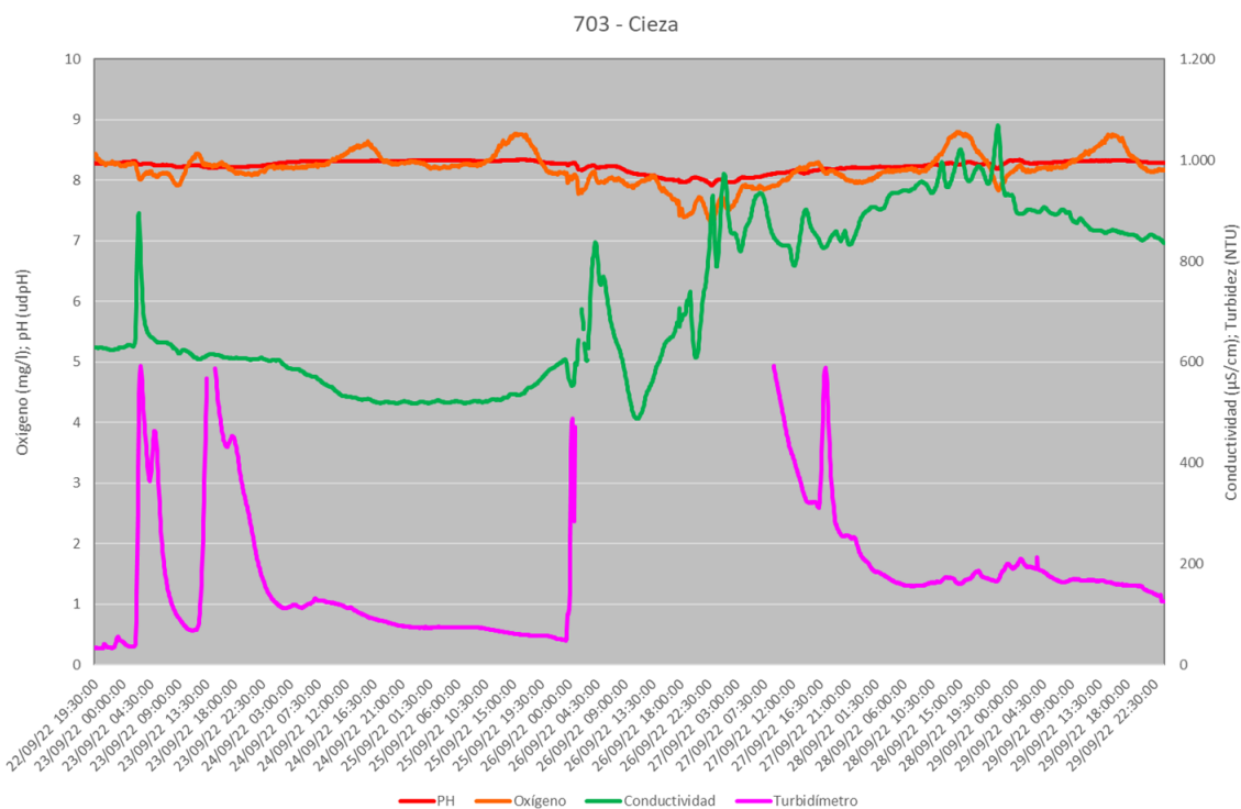
Gráfica 4. Evolución de parámetros en la EA de Cieza: 22 al 29 de septiembre.
