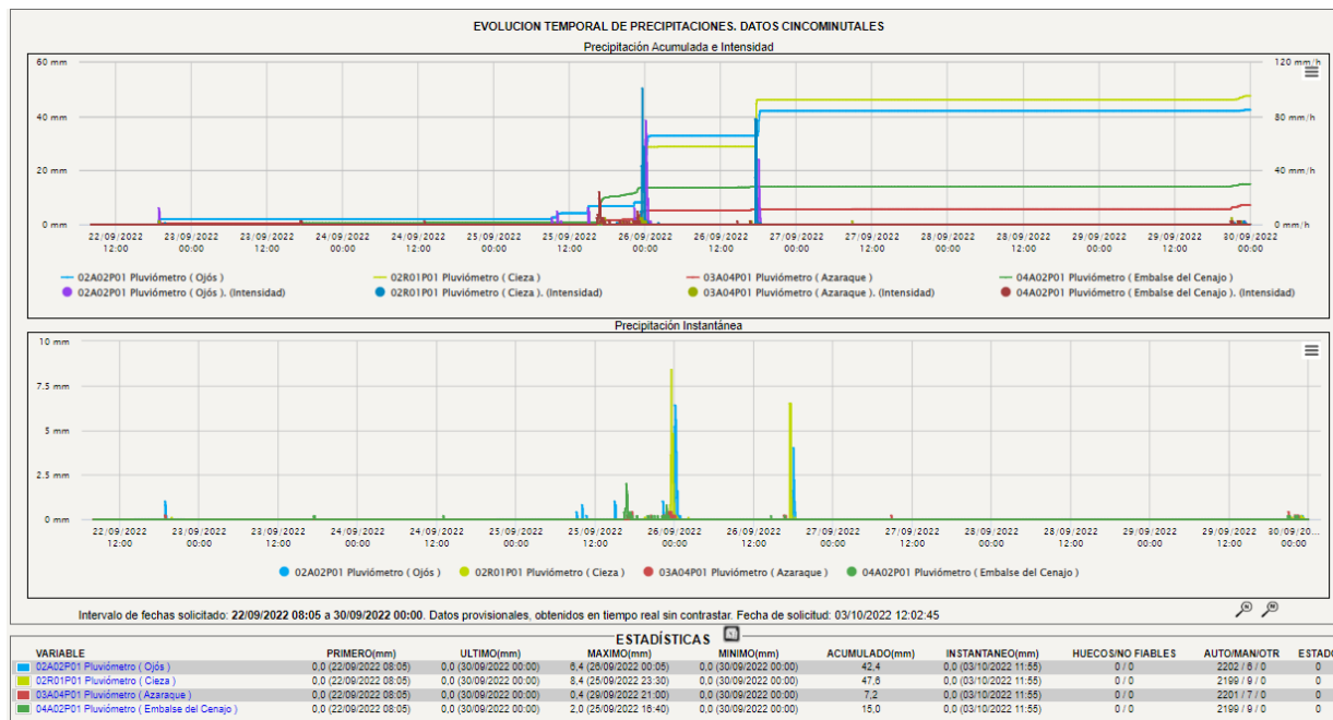
Gráfica 9. Precipitaciones acumuladas durante el episodio: 22 al 29 de septiembre.
