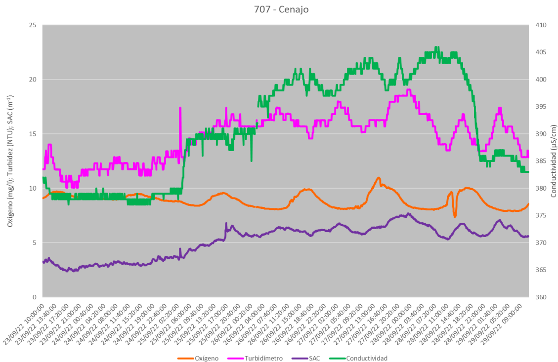
Gráfica 3. Evolución de parámetros en la EA de Cenajo: 23 al 29 de septiembre.
