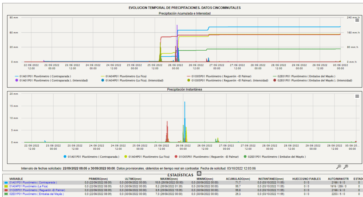
Gráfica 10. Precipitaciones acumuladas durante el episodio: 22 al 29 de septiembre.
