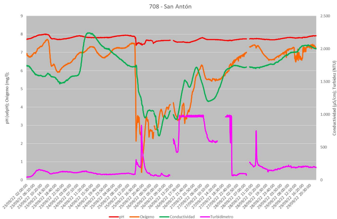
Gráfica 8. Evolución de parámetros en la EA de San Antón: 23 al 29 de septiembre.
