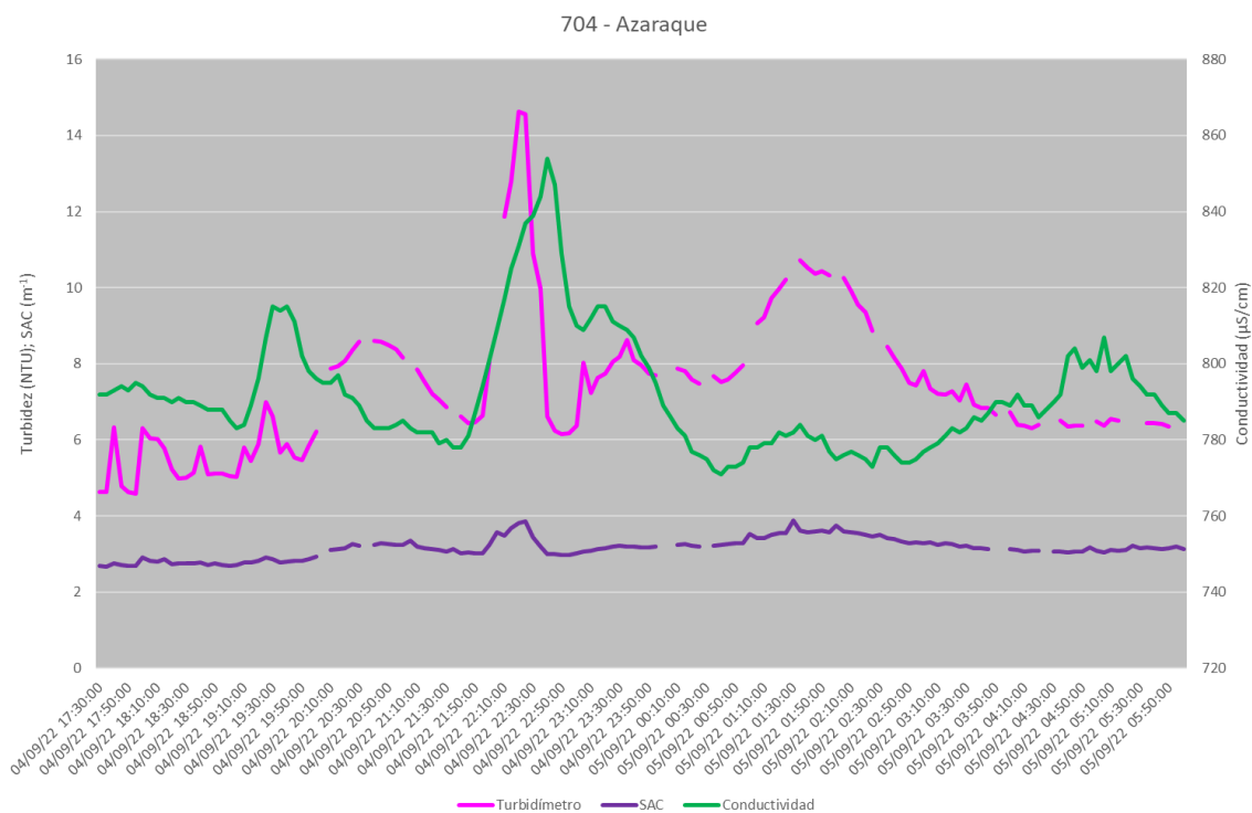
Gráfica 1. Evolución de parámetros en la EA de Azaraque: 4 al 5 de septiembre.
