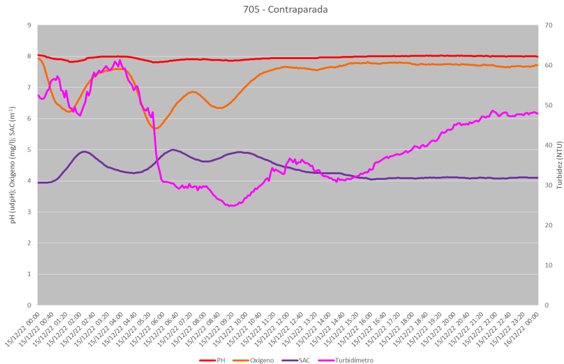
Gráfica 3. Evolución de parámetros en la EA de Contraparada: 15 de diciembre.
