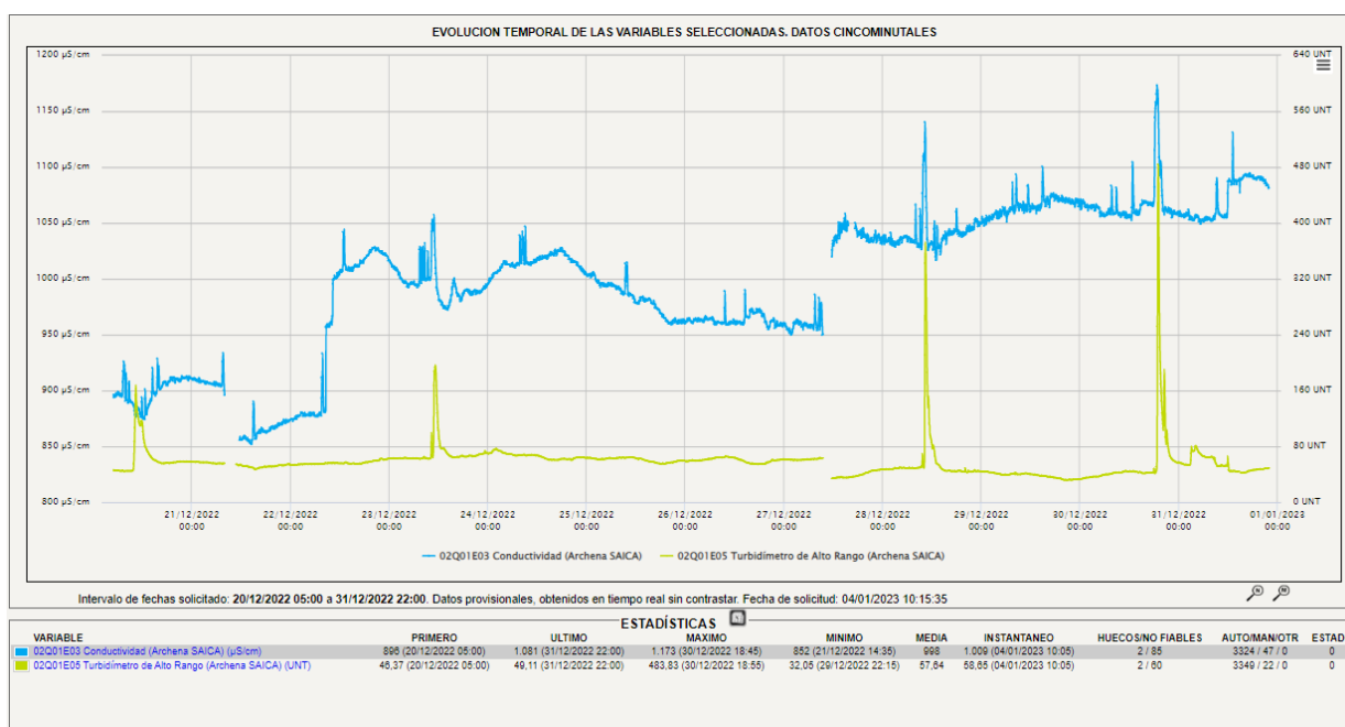
Gráfica 2. Evolución de parámetros en la EA de Archena: 20 al 31 de diciembre.
