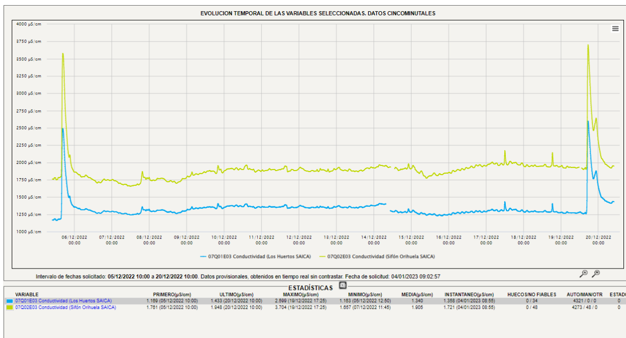
Gráfica 8. Evolución de parámetros en la EA del Sifón de Orihuela: 5 al 20 de diciembre.
