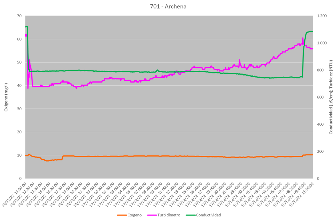
Gráfica 1. Evolución de parámetros en la EA de Archena: 16 al 18 de diciembre.
