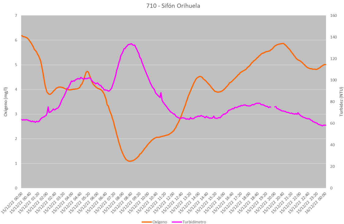
Gráfica 7. Evolución de parámetros en la EA del Sifón de Orihuela: 15 de diciembre.
