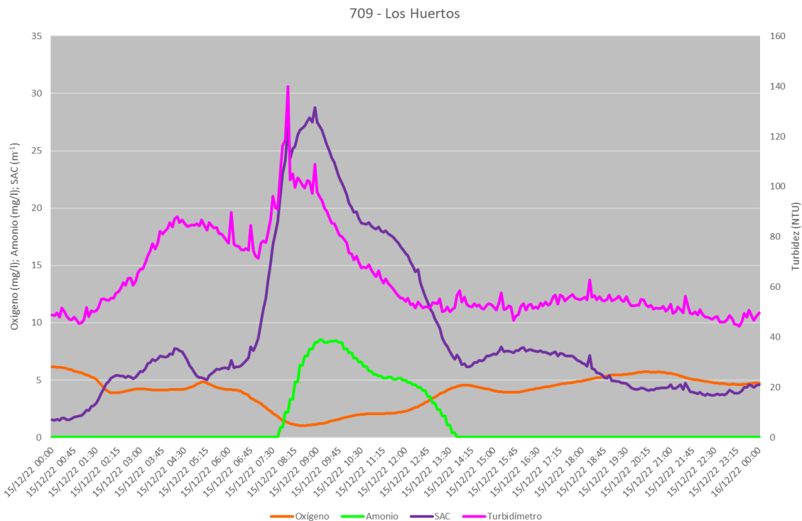
Gráfica 5. Evolución de parámetros en la EA de Los Huertos: 15 de diciembre.
